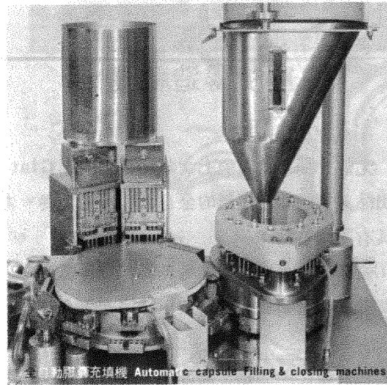
全自動膠囊充填機 Automatic capsule filling & closing machines
