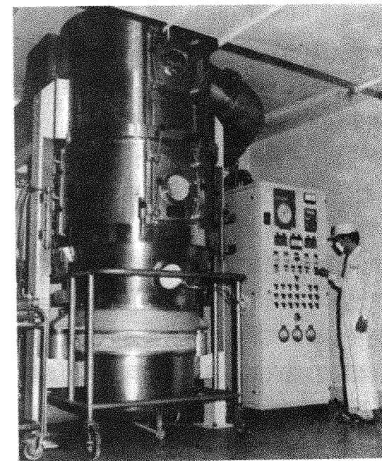
自動噴霧造粒機
