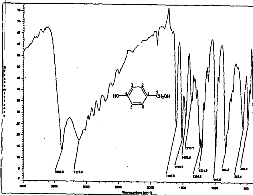
圖十六 天麻苷元 IR (KBr)圖譜
