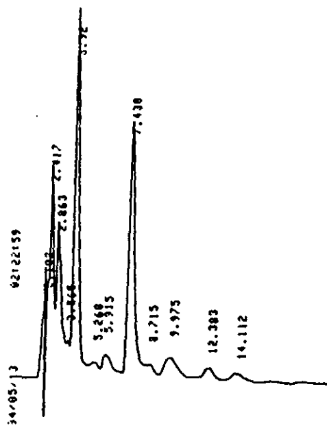
圖三 天麻HPLC層析圖
