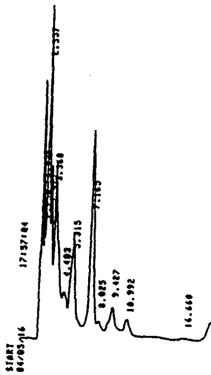
圖六 小兒驚風藥第三方HPLC層析圖
