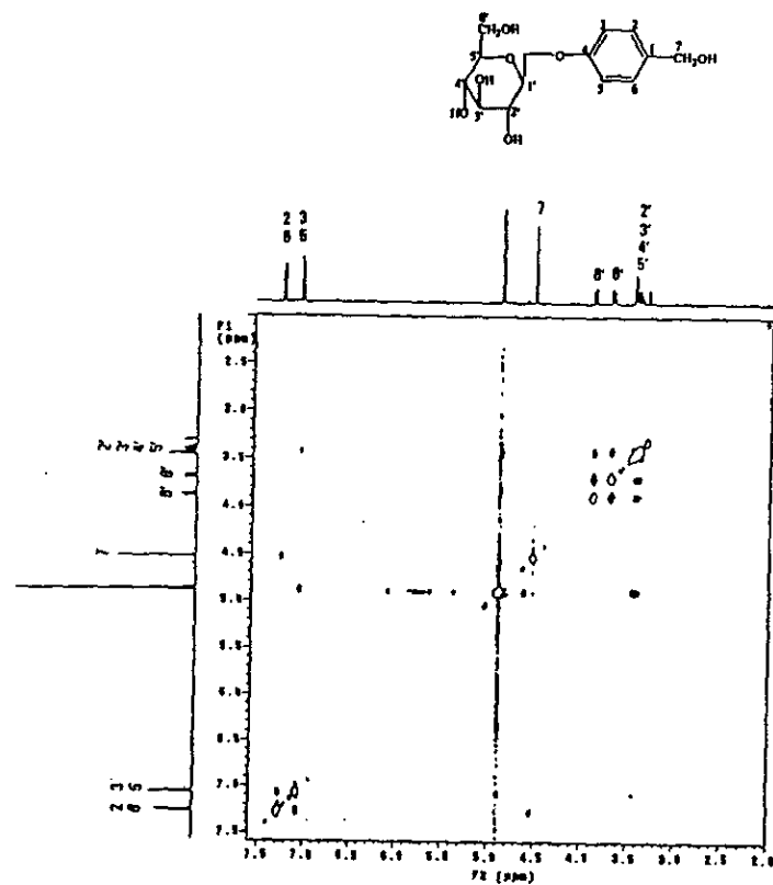
圖十五 天麻素 2D NOSY (CD 3 OD)圖譜
