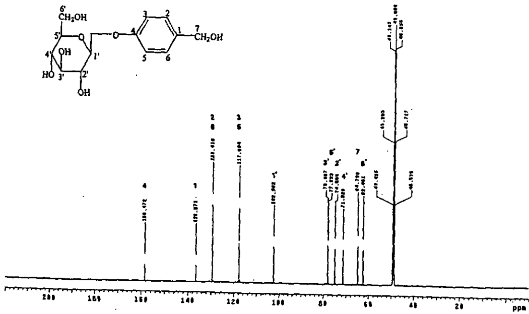
圖十 天麻素 13 C-NMR (CD 3 OD)圖譜
