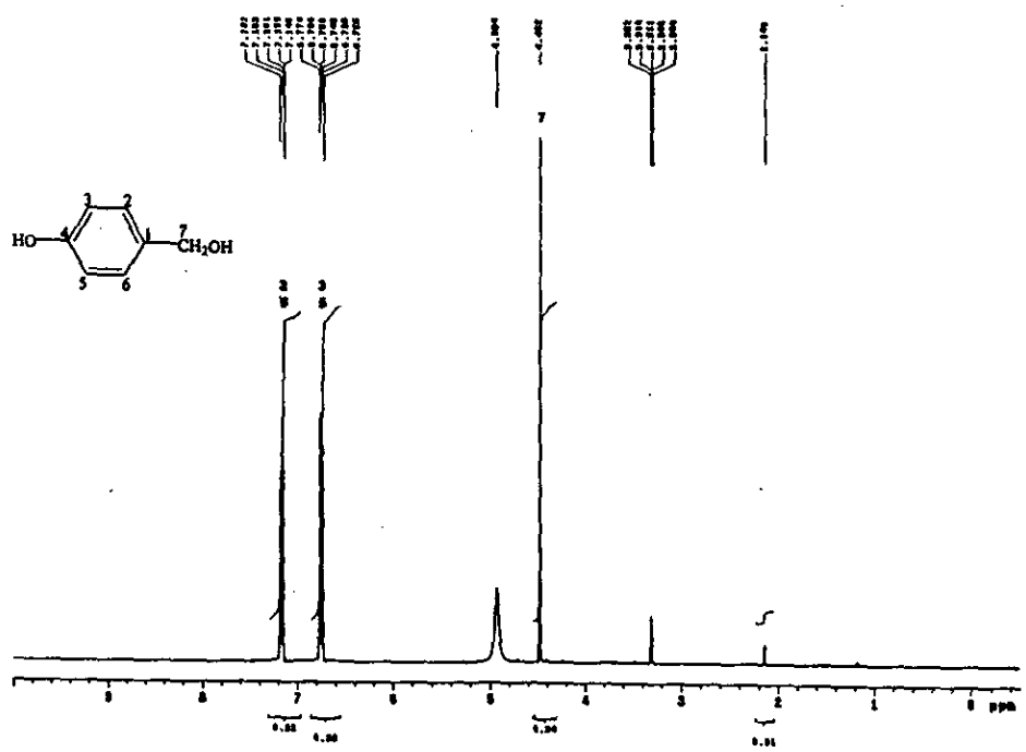
圖十八 天麻苷元 1 H-NMR (CD 3 OD)圖譜
