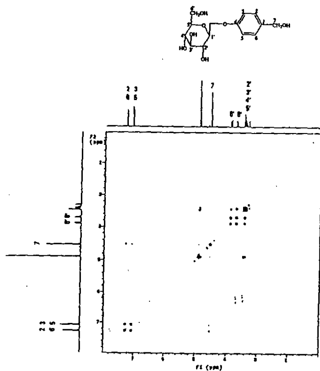
圖十二 天麻素 2D 1 H- 1 H COSY (CD 3 OD)圖譜
