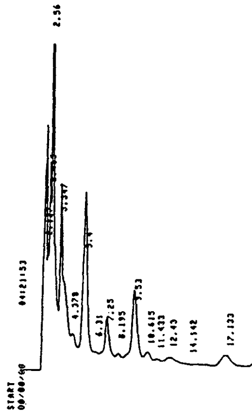
圖五 半夏白朮天麻湯HPLC層析圖
