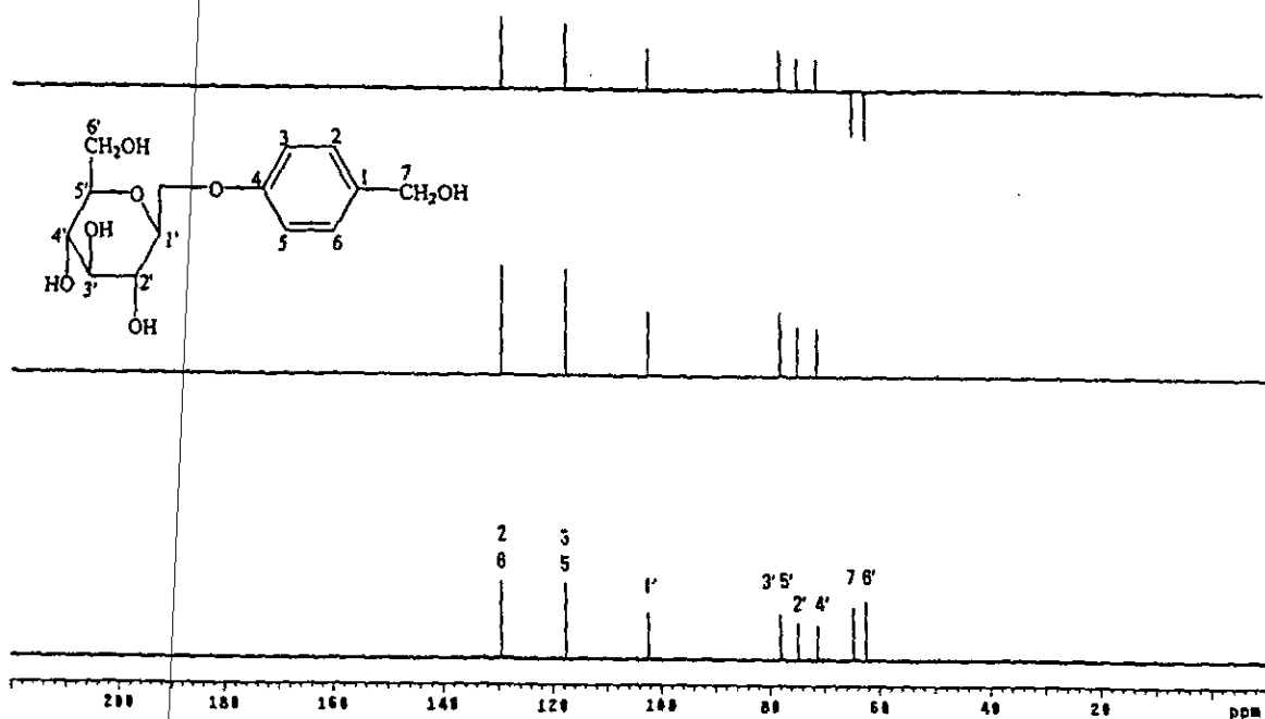
圖十一 天麻素 DEPT (CD 3 OD)圖譜
