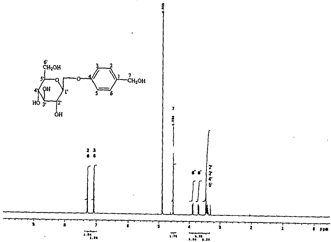
圖九 天麻素 1 H-NMR (CD 3 OD)圖譜
