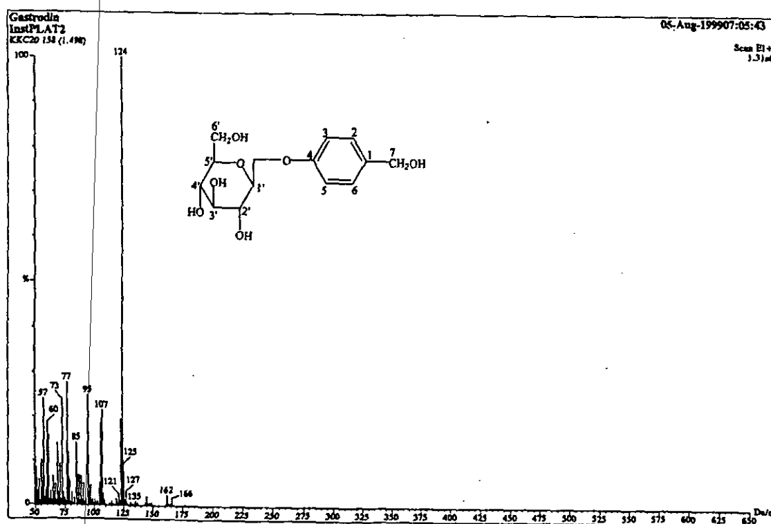
圖八 天麻素 Mass (EI)圖譜
