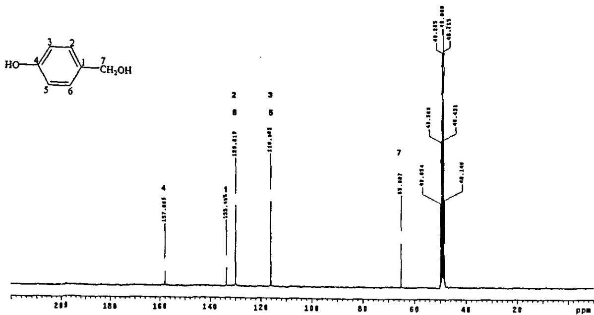
圖十九 天麻苷元 ^{13}\text{C} -NMR ( \text{CD}_3\text{OD} )圖譜
