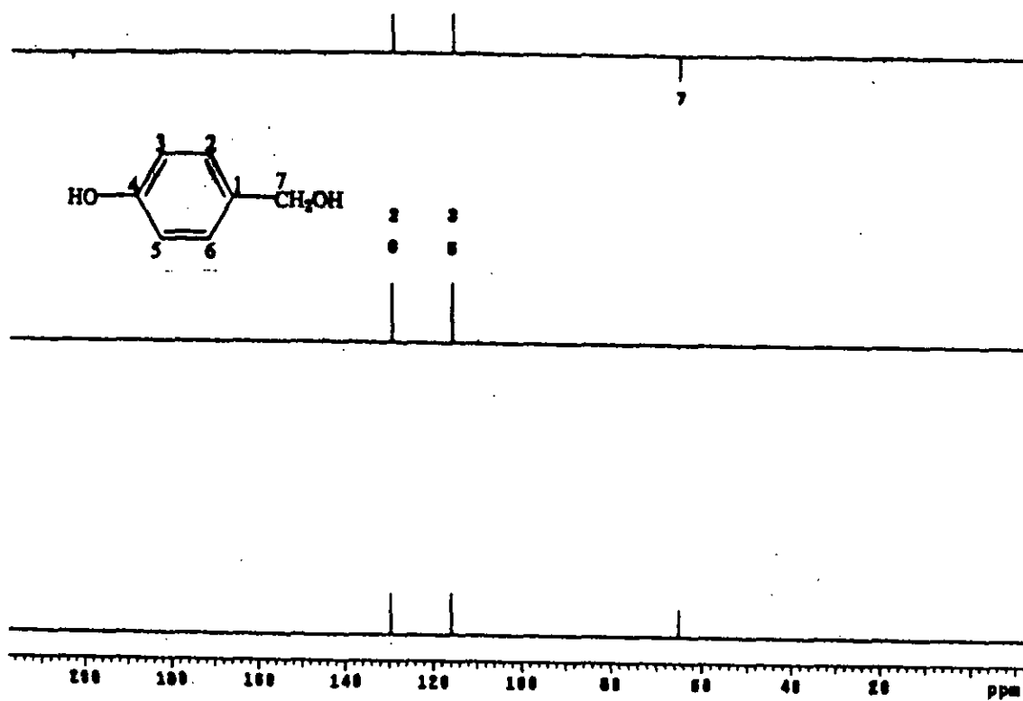
圖二十 天麻苷元 DEPT ( \text{CD}_3\text{OD} )圖譜
