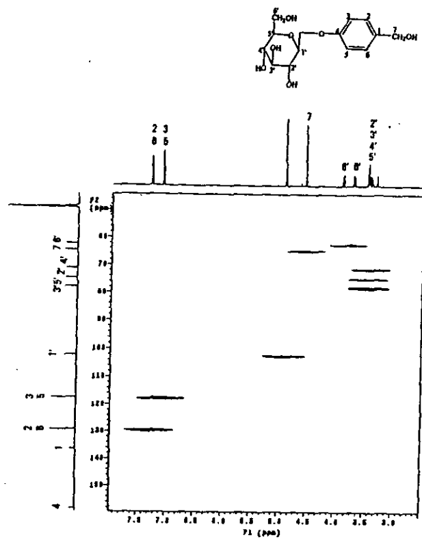
圖十三 天麻素 2D HMQC (CD 3 OD)圖譜
