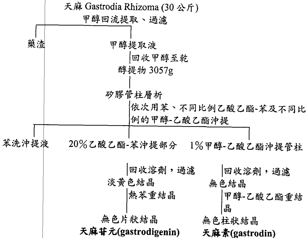
圖二 天麻( Gastrodia elata Blume)塊莖之抽提流程圖
