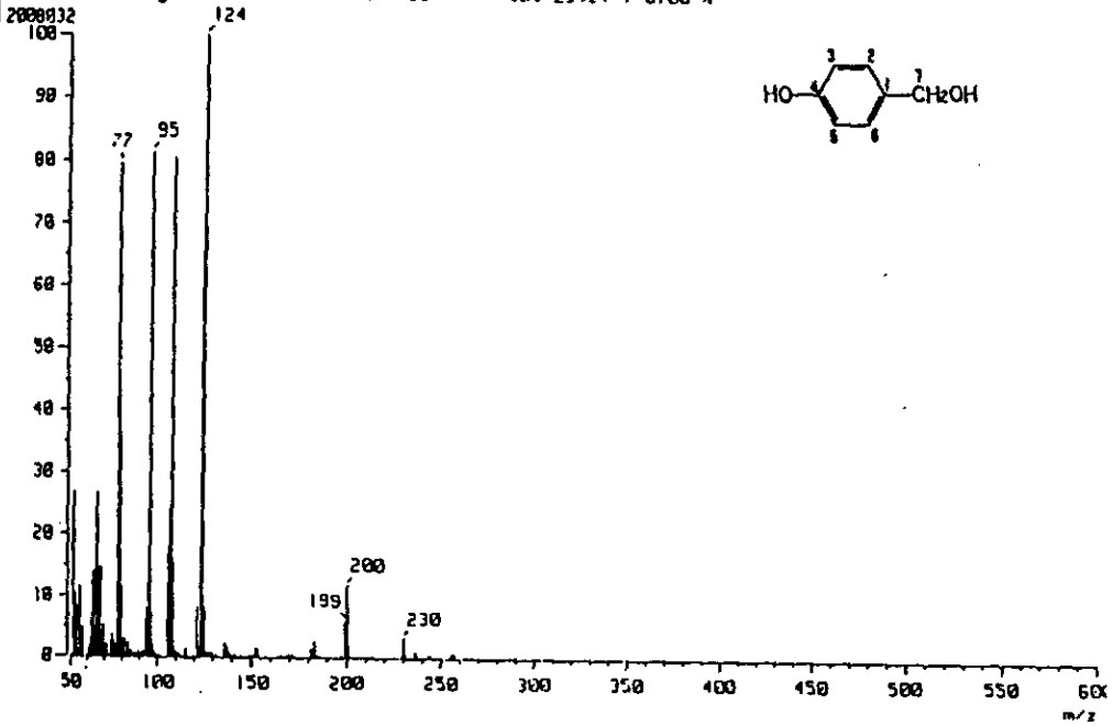
圖十七 天麻苷元 Mass (EI)圖譜
