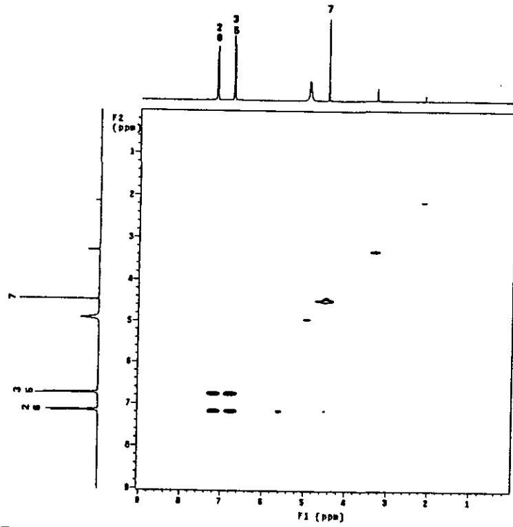
圖廿一 天麻昔元 2D 1 H- 1 H COSY (CD 3 OD)圖譜
