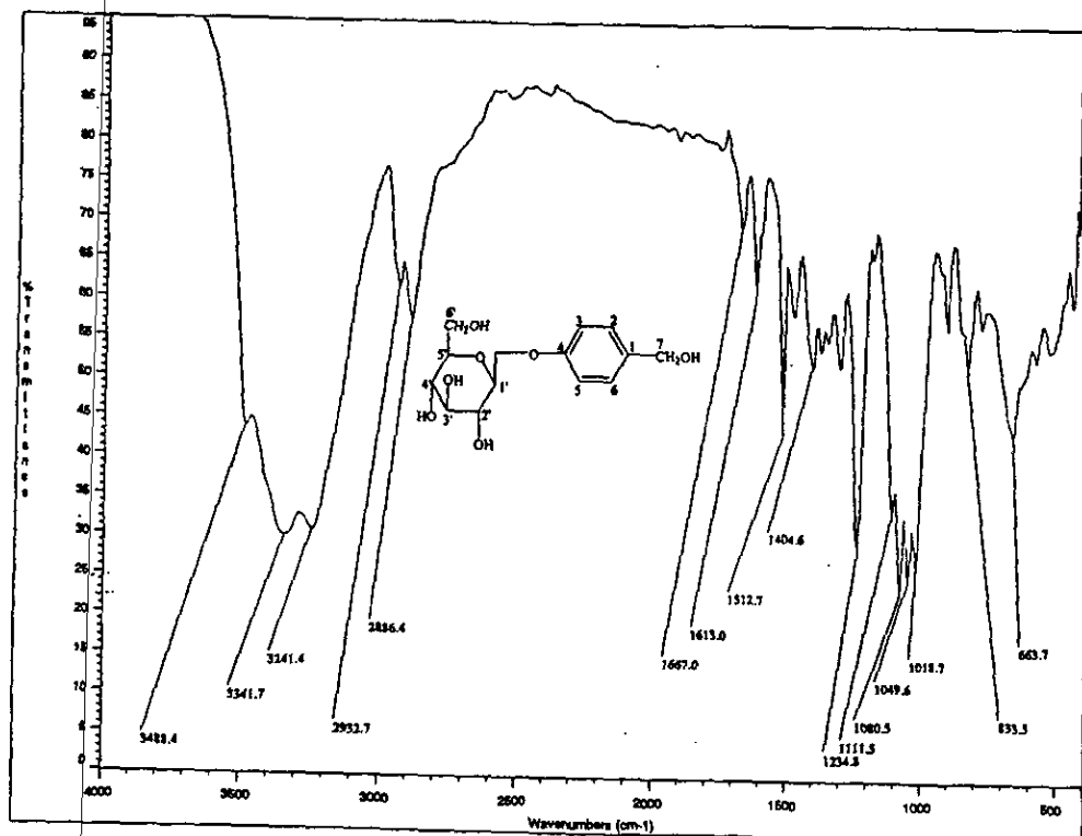
圖七 天麻素 IR (KBr)圖譜
