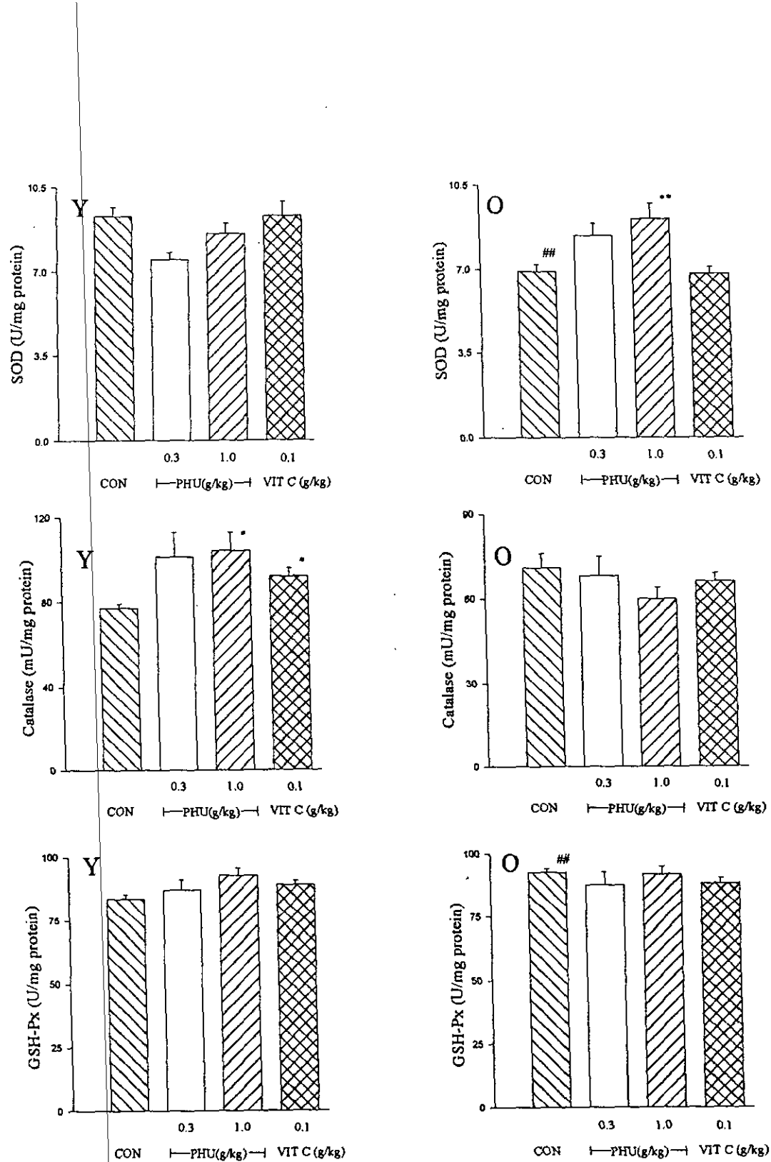
圖三、人尿製備物對大鼠腦部抗氧化酵素活性的影響
