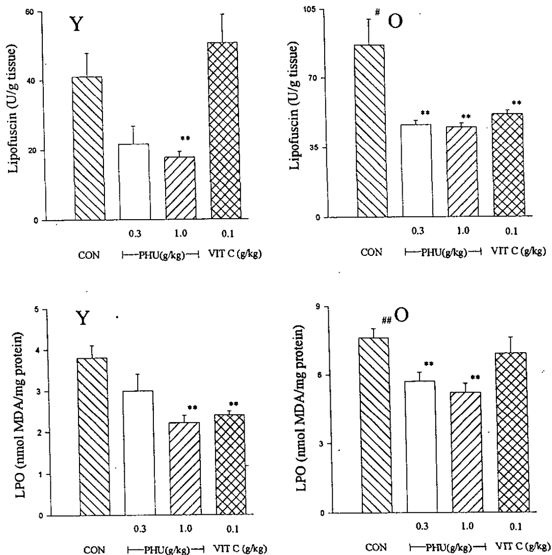
圖二、人尿製備物對大鼠腦部脂質過氧化及脂褐素的影響 Y：年輕大鼠； O：中老年大鼠； LPO：脂質過氧化； Lipofuscin：脂褐素 All values are means \pm S.E. * p < 0.05 , ** p < 0.01 compared with respect control group. # p < 0.05 , ## p < 0.01 compared with young control group.
