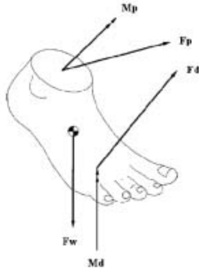
圖 2.4 自由體圖
