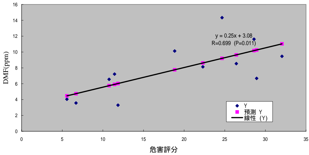
圖三、三家合成皮工廠十二個相似暴露群空氣中DMF濃度與危害評分線性迴歸圖
