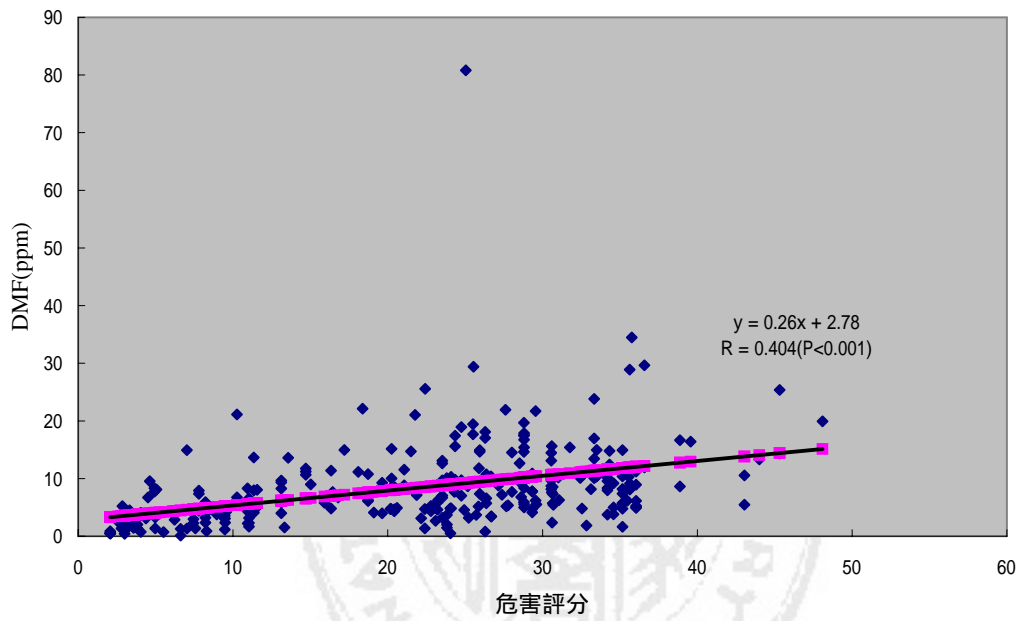
圖四、三家合成皮工廠受測樣本DMF濃度與危害評分之線性迴歸方程式
