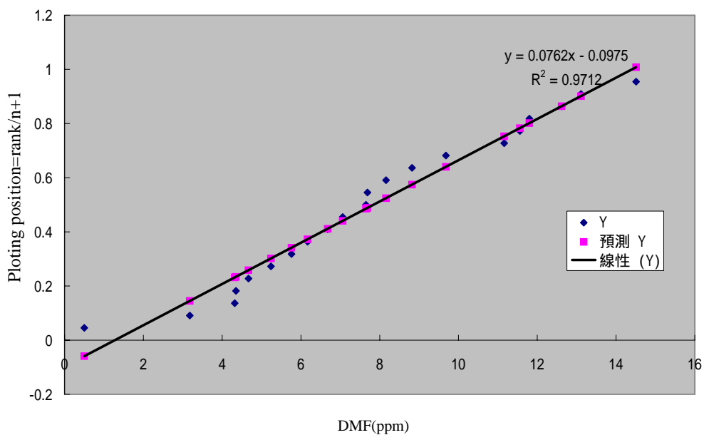
圖一、檢定A工廠SEG1環測DMF濃度之線性迴歸圖
