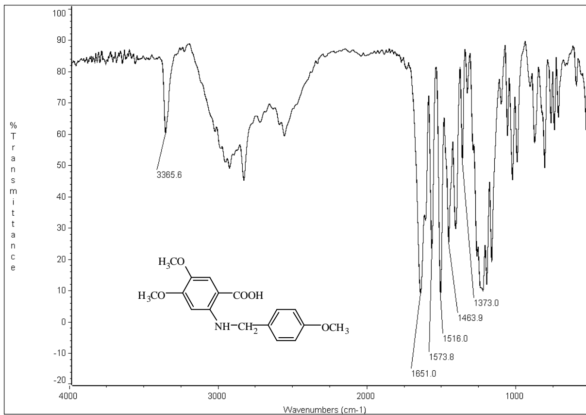
圖 75-2 IR (KBr) spectrum of compound 75
