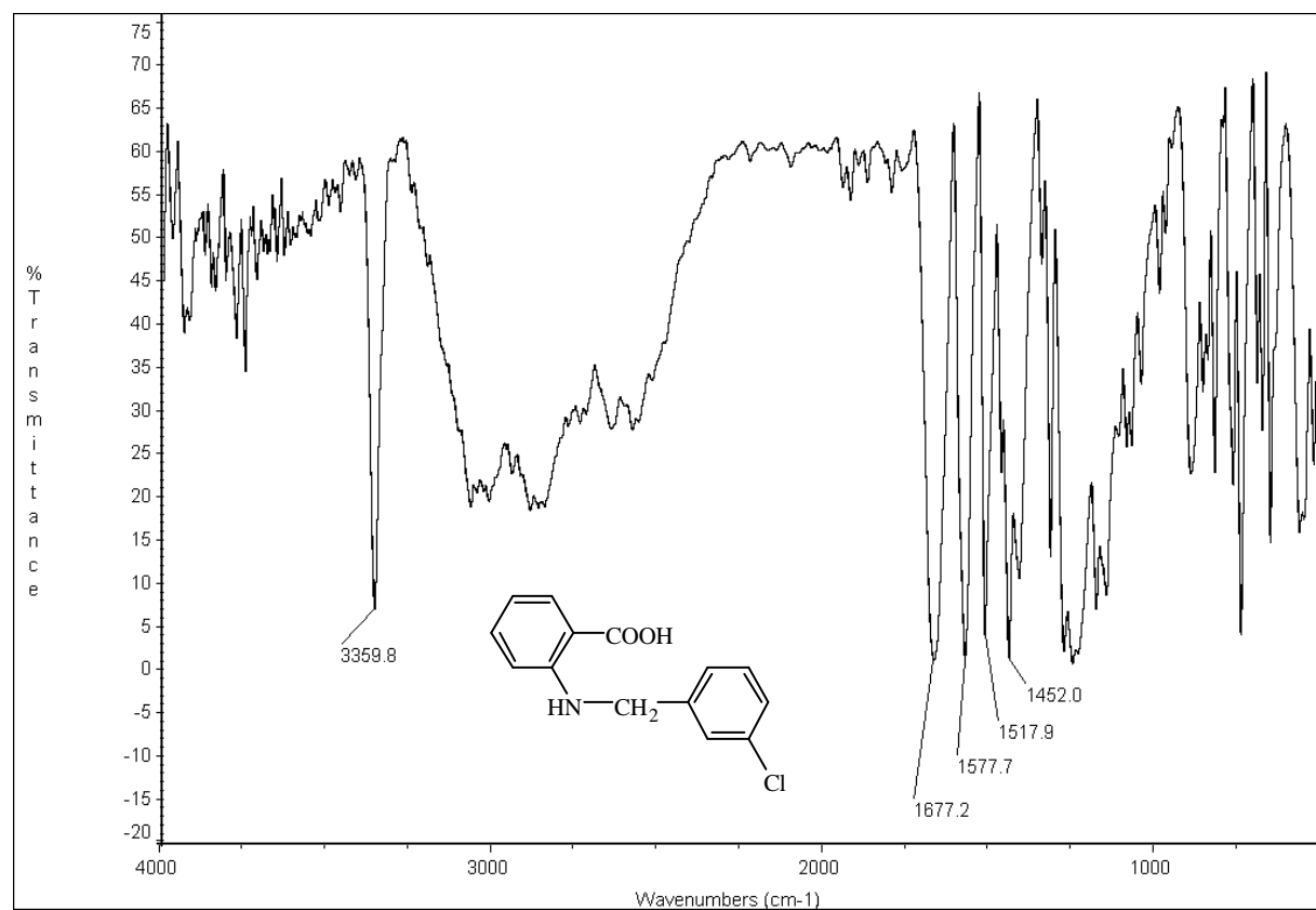
圖 67-2 IR (KBr) spectrum of compound 67
