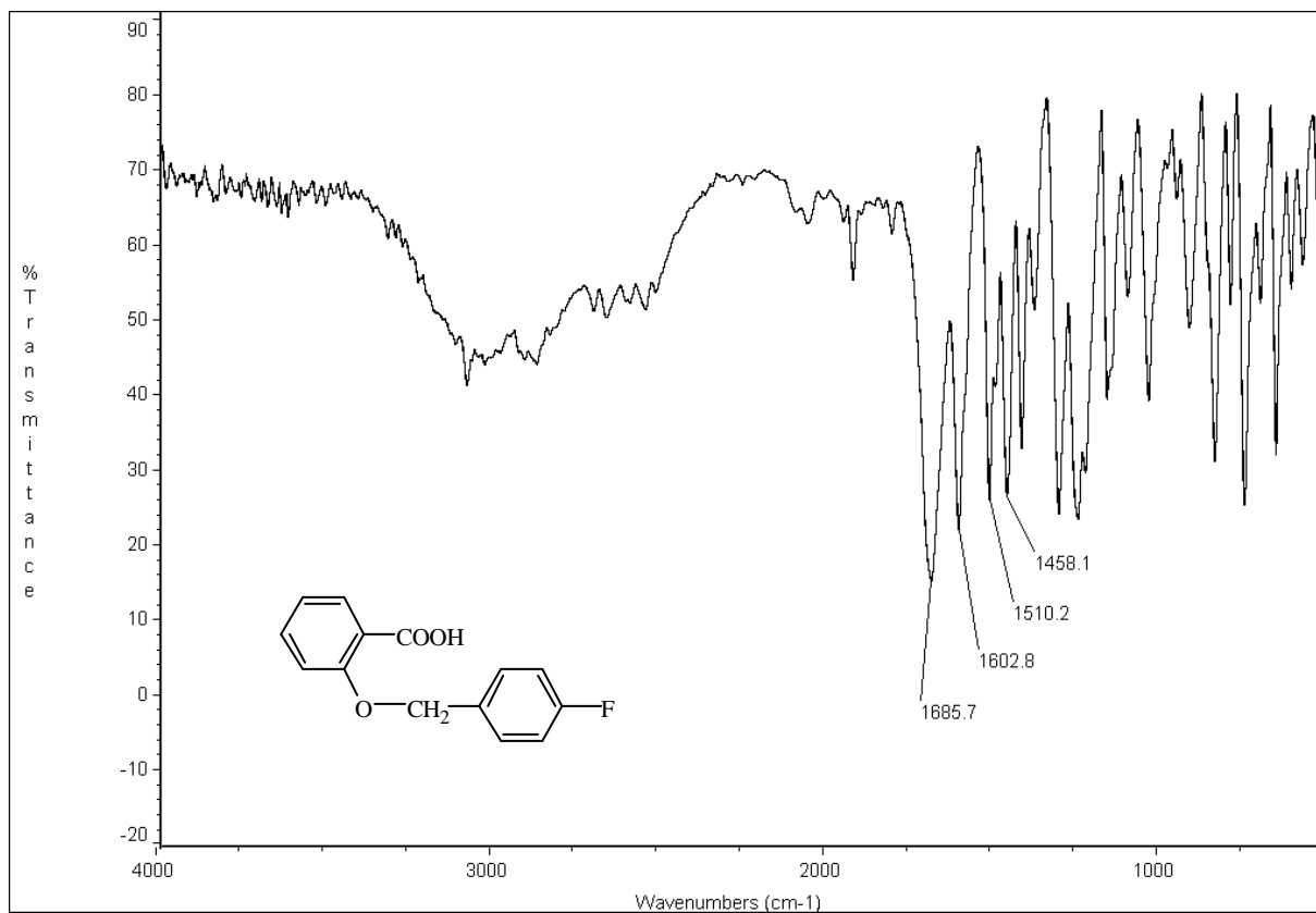
圖 62-2 IR (KBr) spectrum of compound 62
