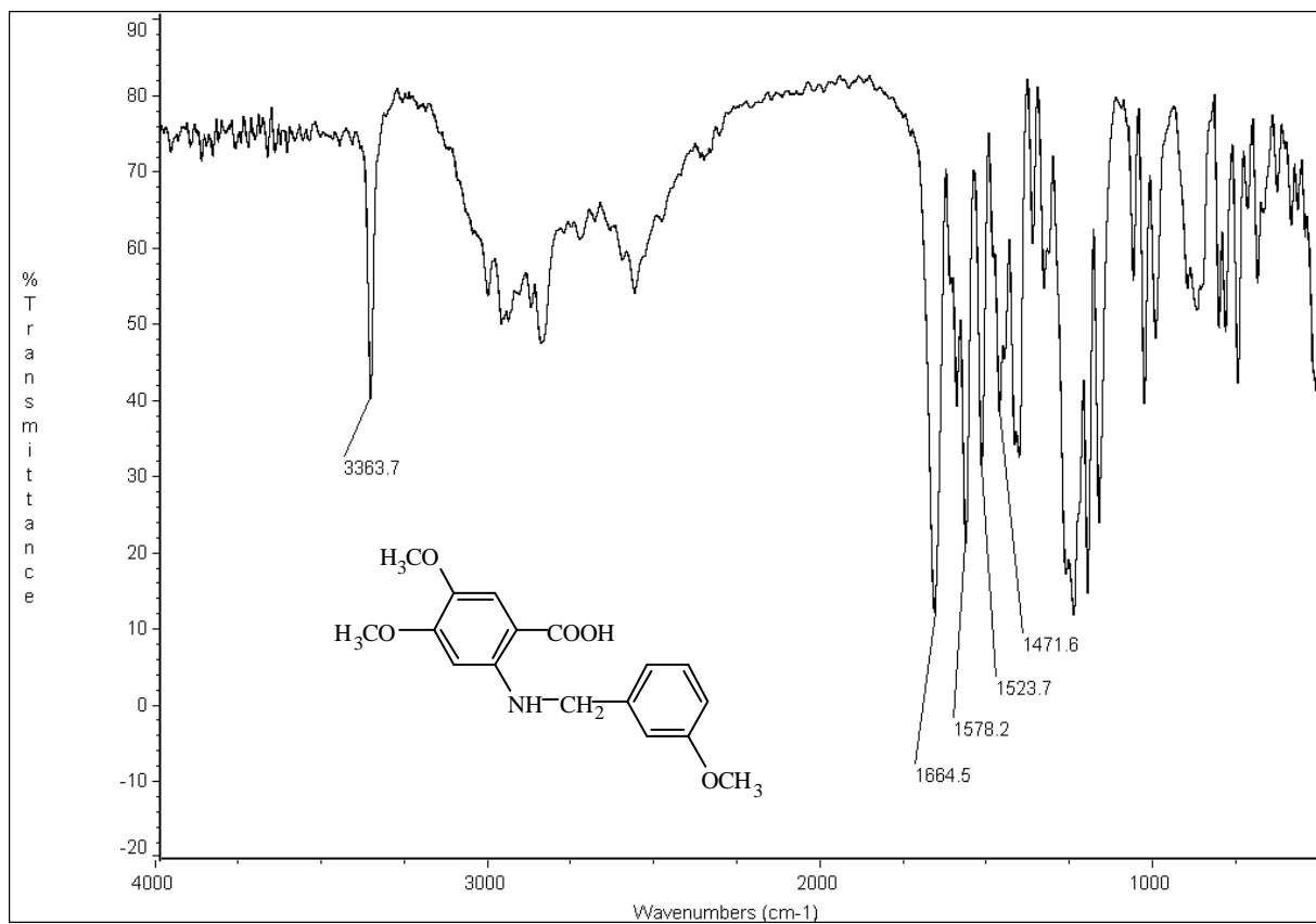
圖 74-2 IR (KBr) spectrum of compound 74
