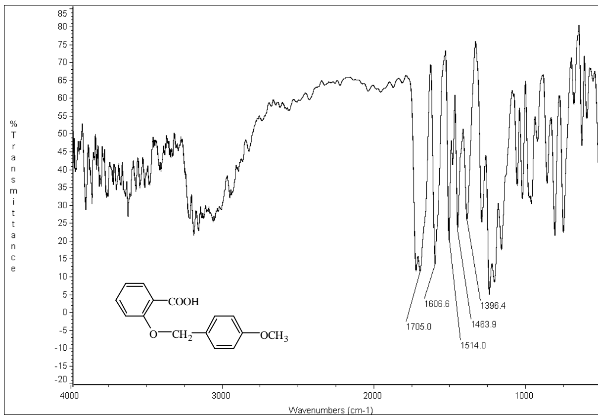
圖 64-2 IR (KBr) spectrum of compound 64
