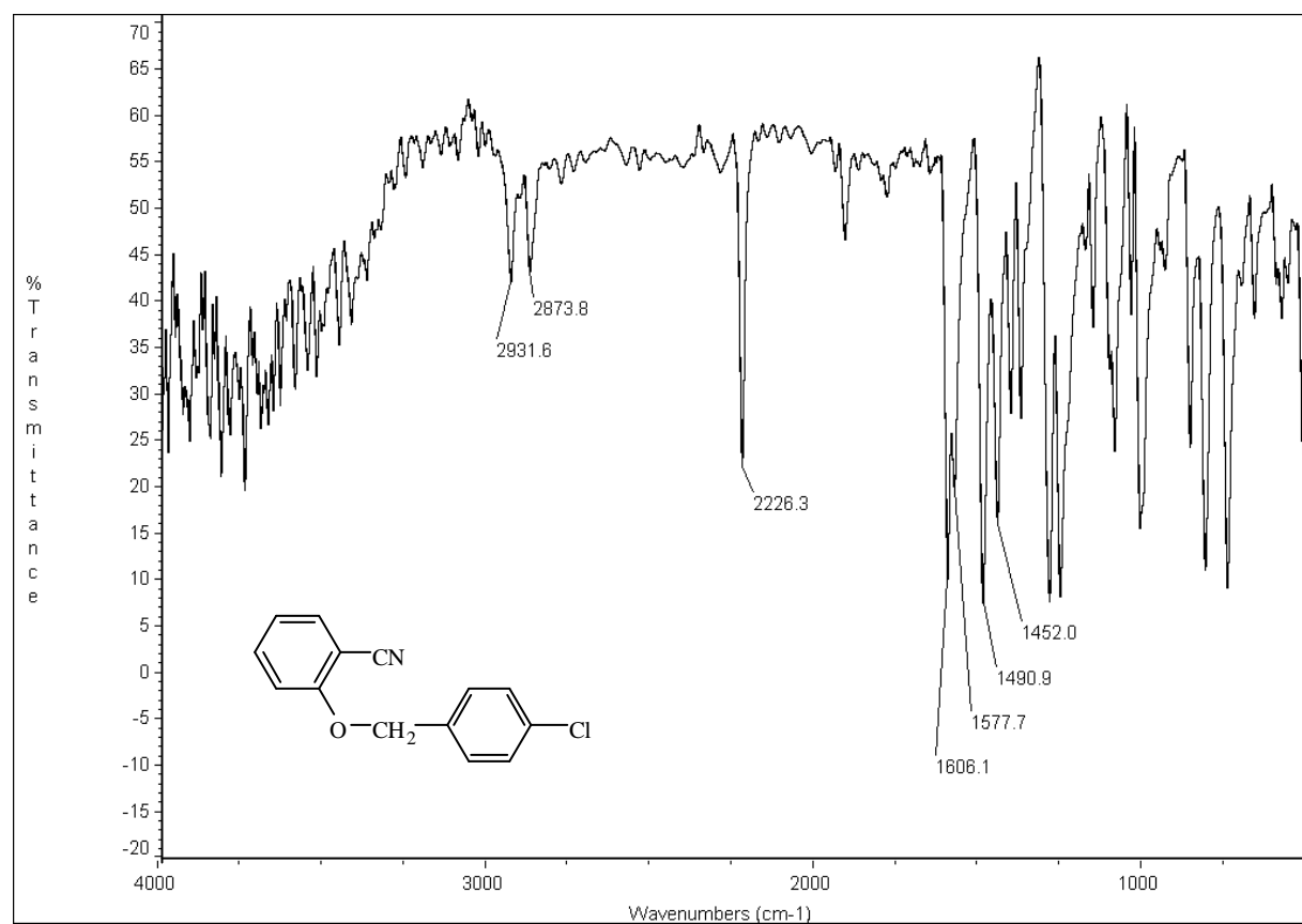
圖 20-2 IR (KBr) spectrum of compound 20
