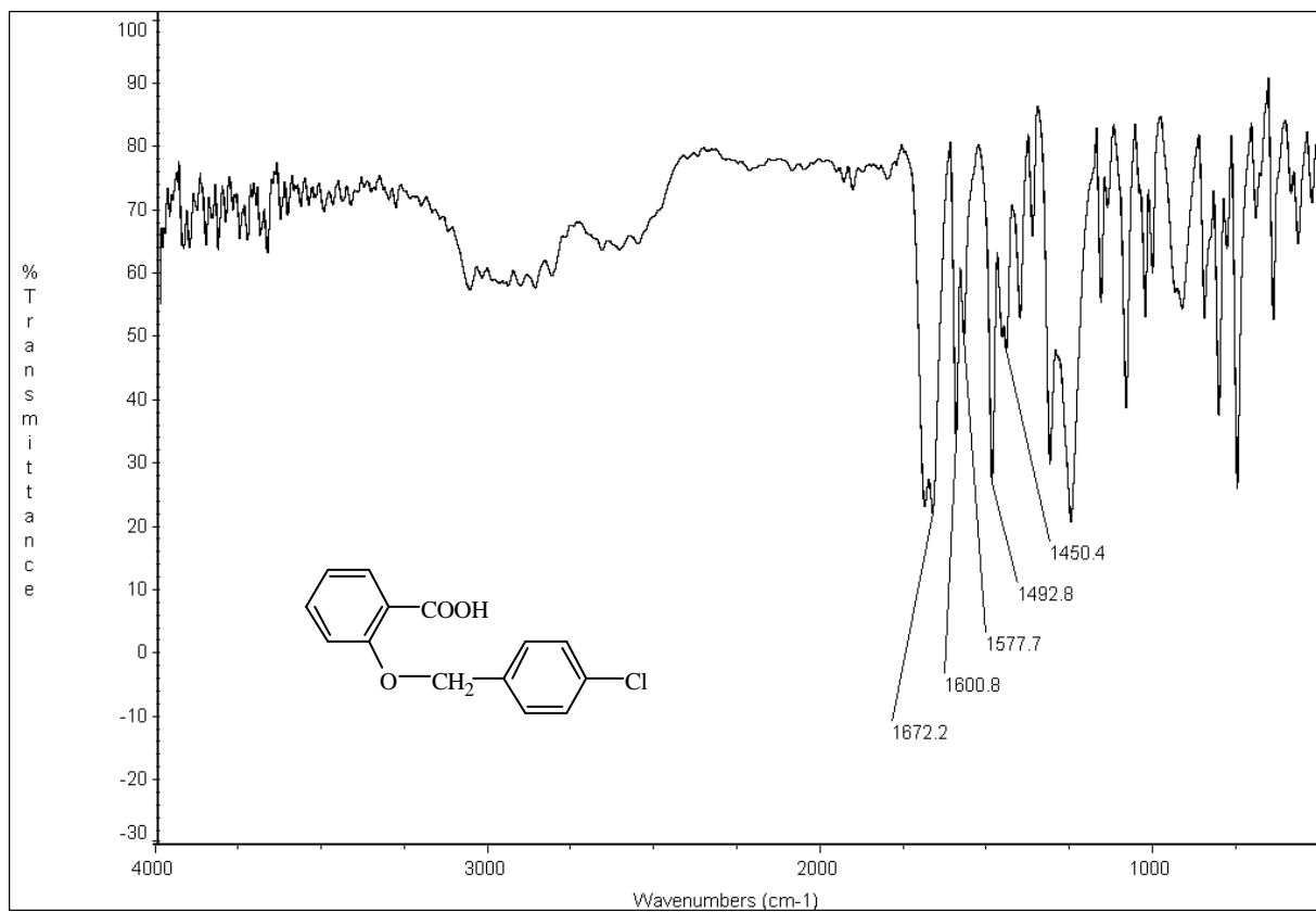
圖 59-2 IR (KBr) spectrum of compound 59
