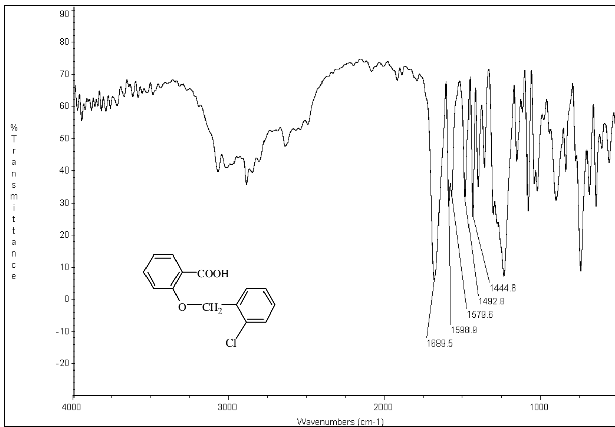
圖 57-2 IR (KBr) spectrum of compound 57
