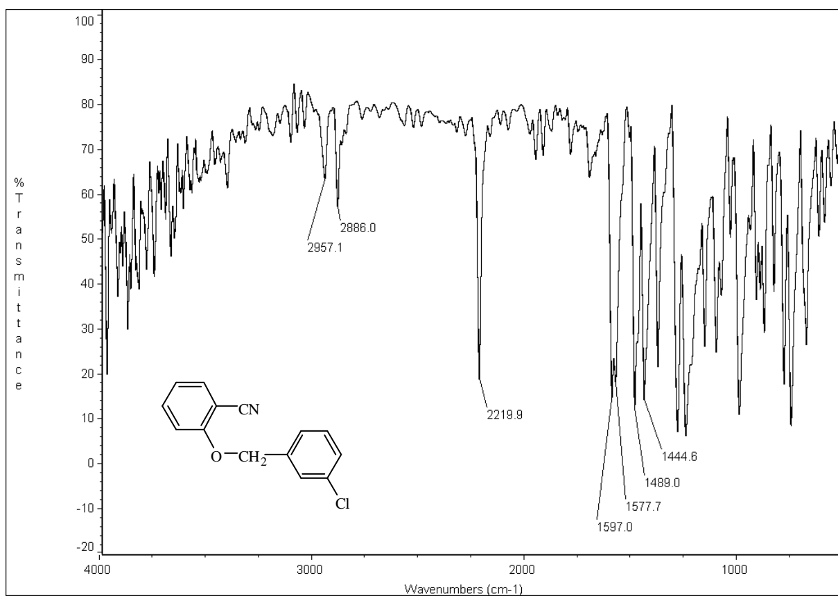
圖 19-2 IR (KBr) spectrum of compound 19
