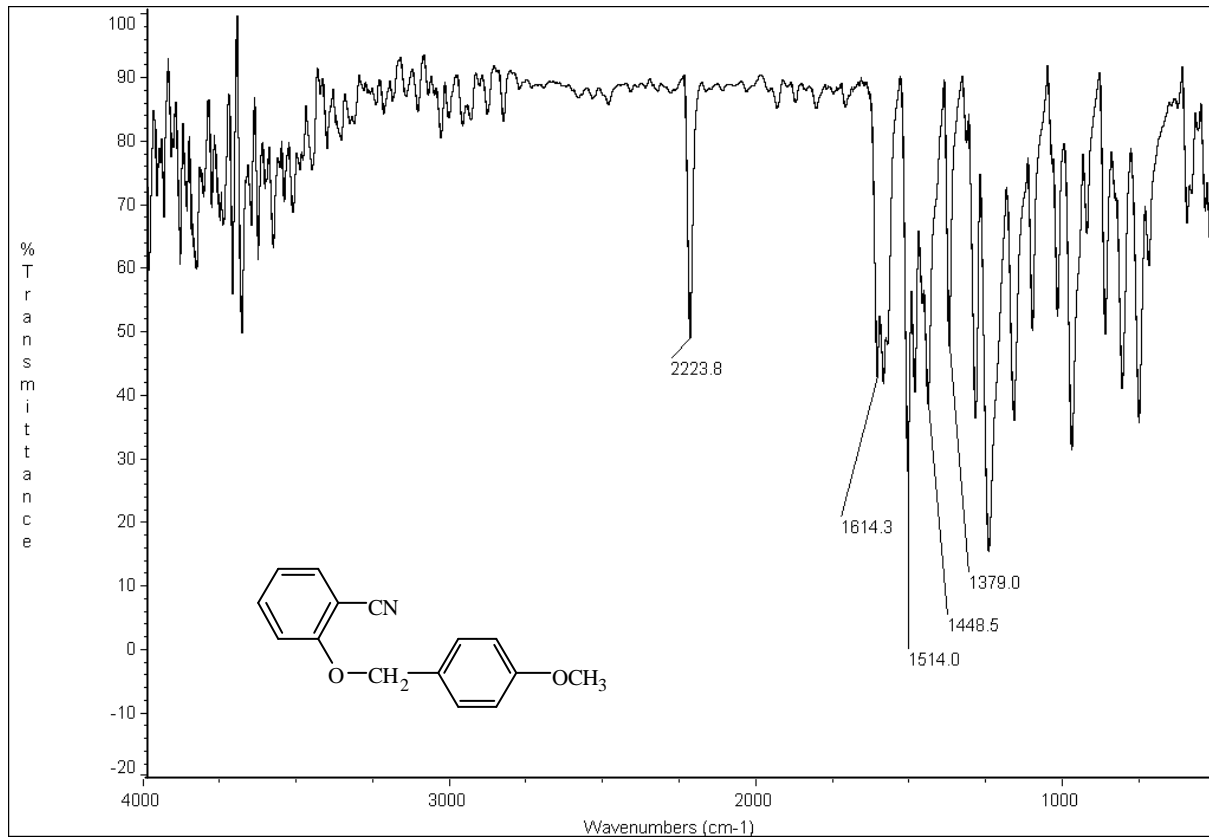
圖 25-2 IR (KBr) spectrum of compound 25
