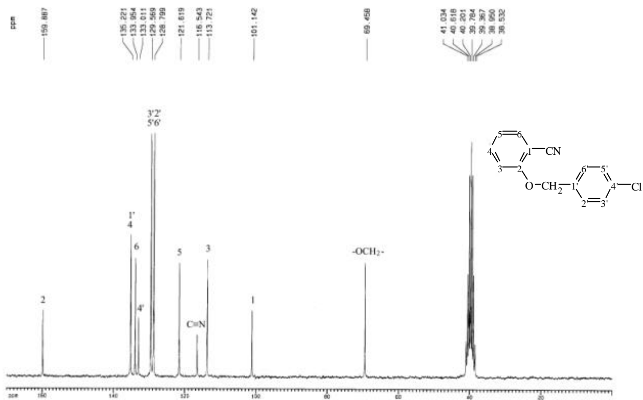
圖 20-4 ^{13}\text{C-NMR} (CDCl 3 , 50 MHz) spectrum of compound 20
