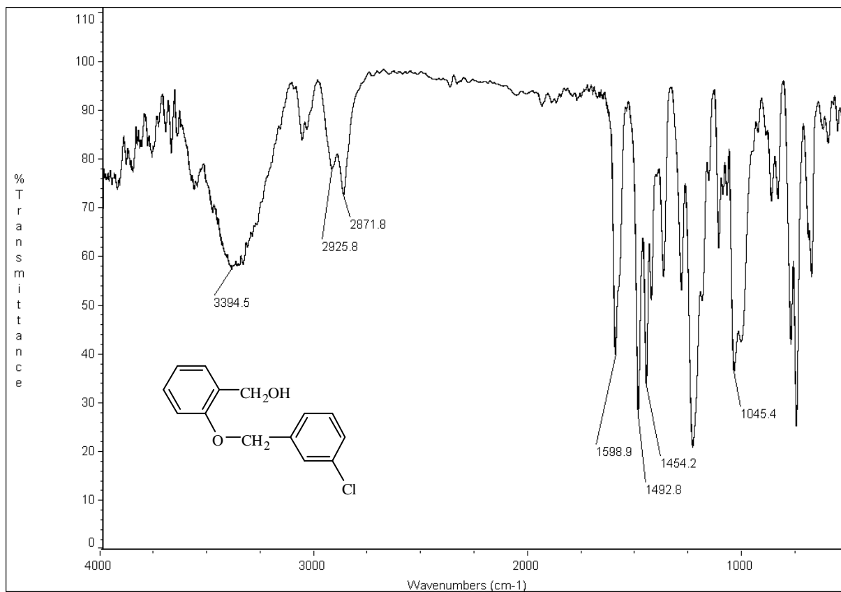
圖 32-2 IR (KBr) spectrum of compound 32
