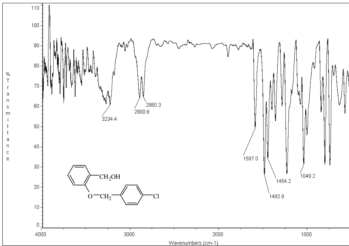
圖 33-2 IR (KBr) spectrum of compound 33
