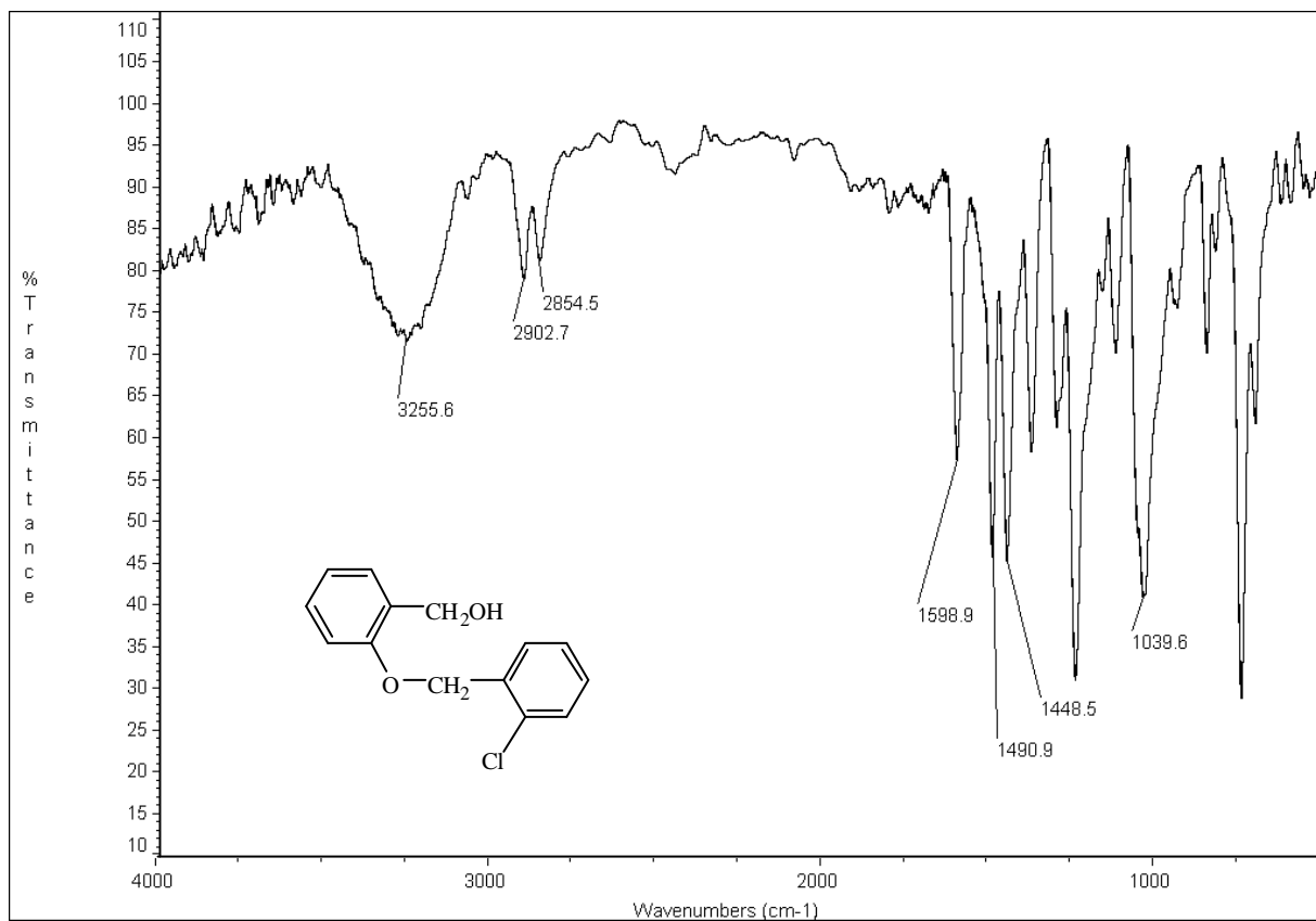
圖 31-2 IR (KBr) spectrum of compound 31
