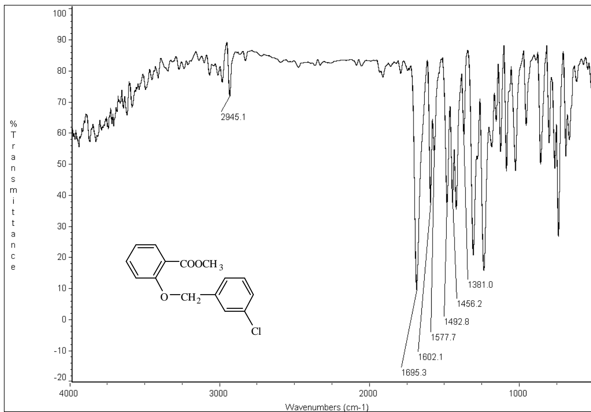
圖 36-2 IR (KBr) spectrum of compound 36
