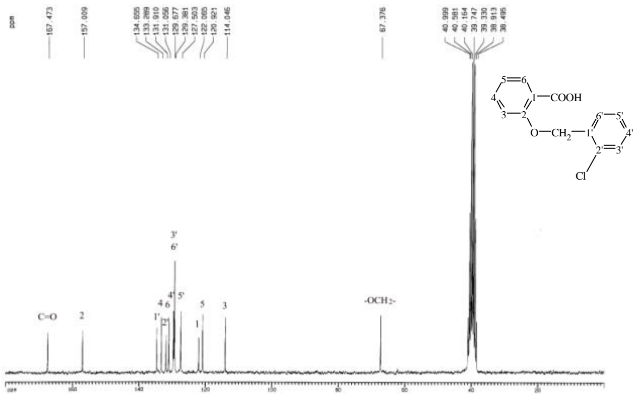
圖 57-4 ^{13}\text{C-NMR} ( \text{DMSO-}d_6 , 50 MHz) spectrum of compound 57
