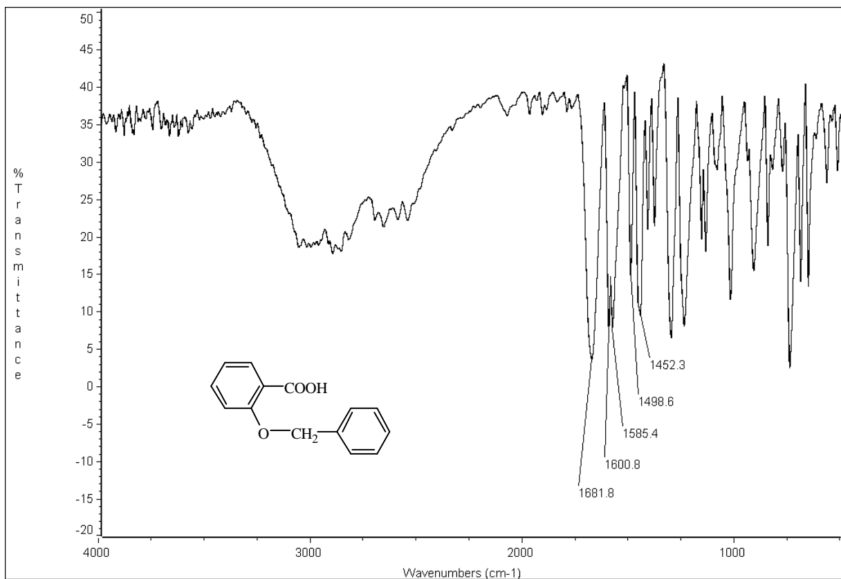
圖 56-2 IR (KBr) spectrum of compound 56
