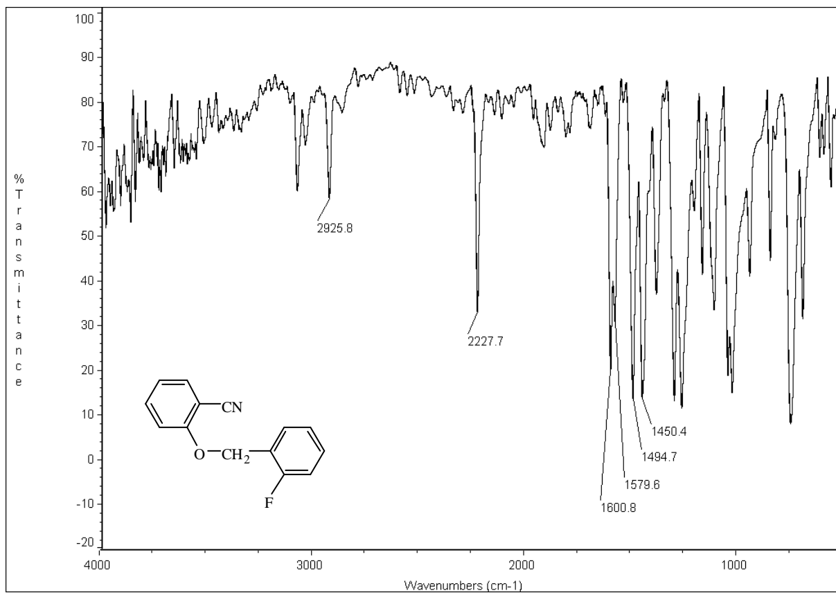
圖 21-2 IR (KBr) spectrum of compound 21
