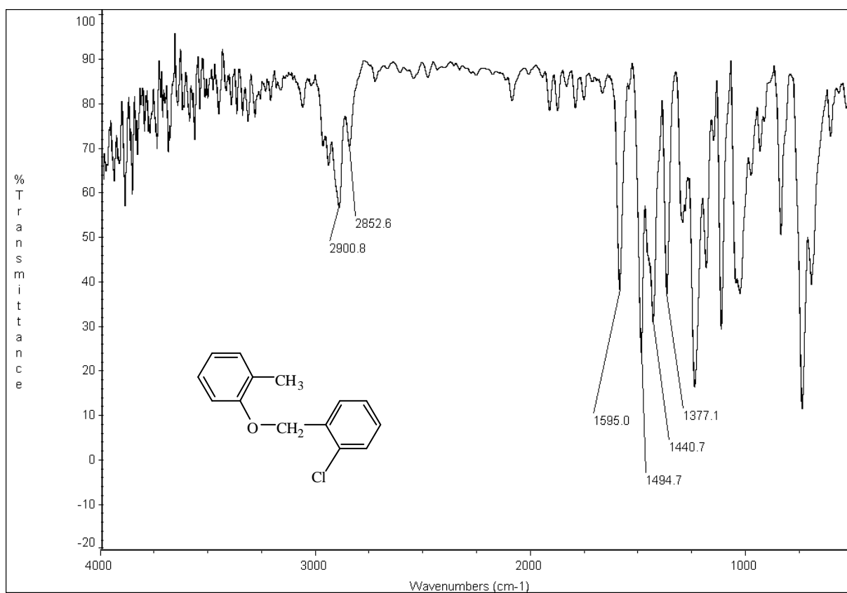
圖 27-2 IR (KBr) spectrum of compound 27
