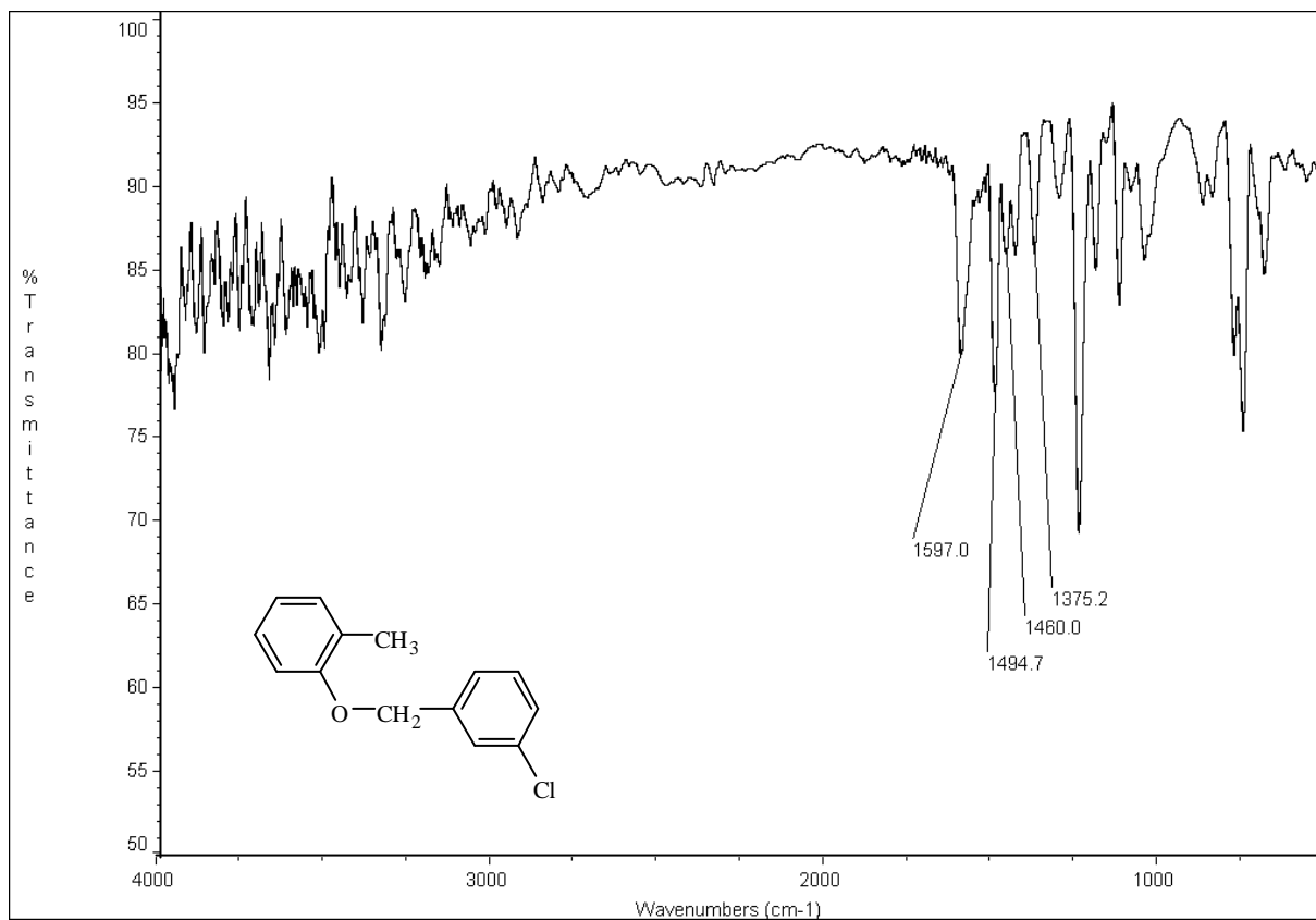
圖 28-2 IR (KBr) spectrum of compound 28
