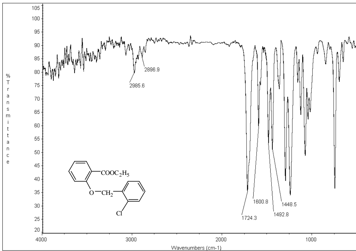
圖 39-2 IR (KBr) spectrum of compound 39
