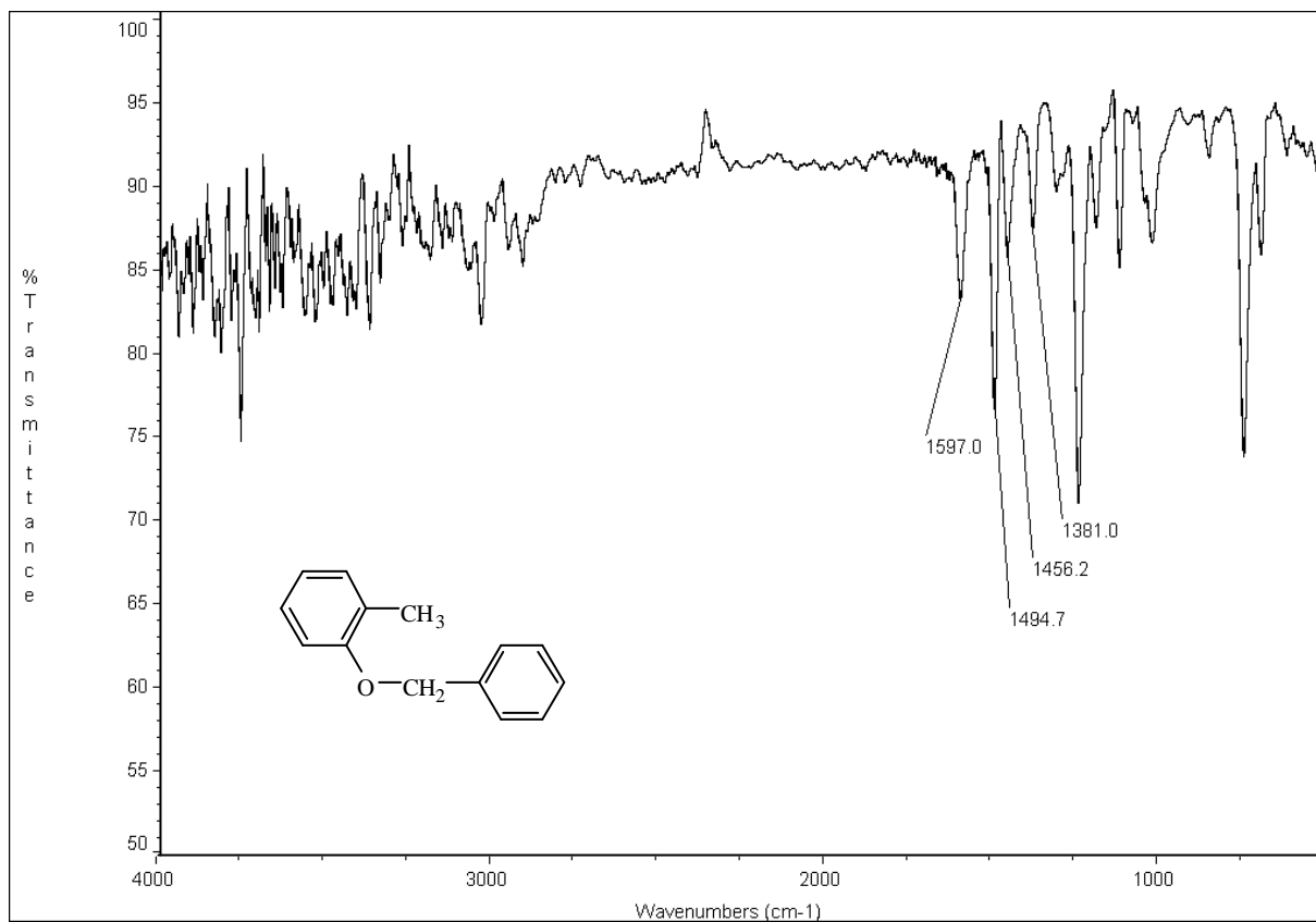
圖 26-2 IR (KBr) spectrum of compound 26
