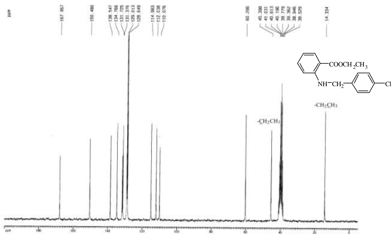
圖 48-2 ^{13}\text{C-NMR} ( \text{DMSO-}d_6 , 50 MHz) spectrum of compound 48
