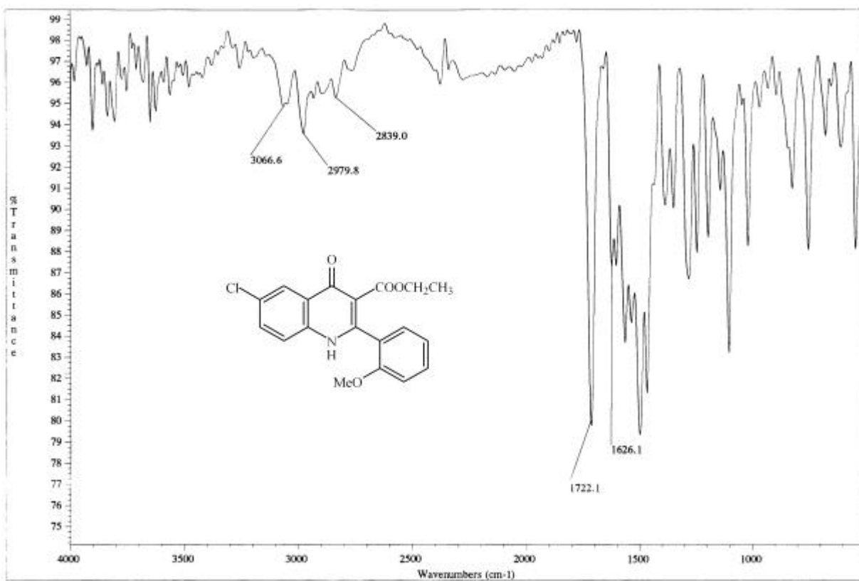
圖 33-2 化合物 33 之 IR 圖譜
