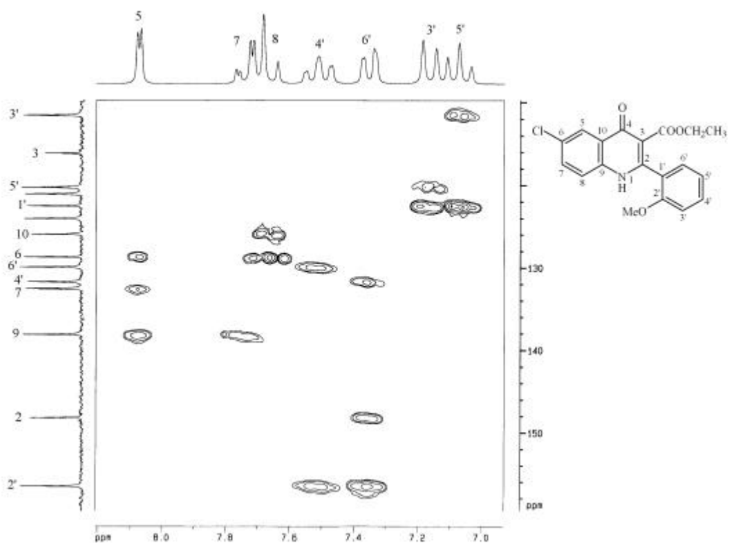
圖 33-10 化合物 33 之 HMBC (DMSO- d 6 , 200 MHz)圖譜
