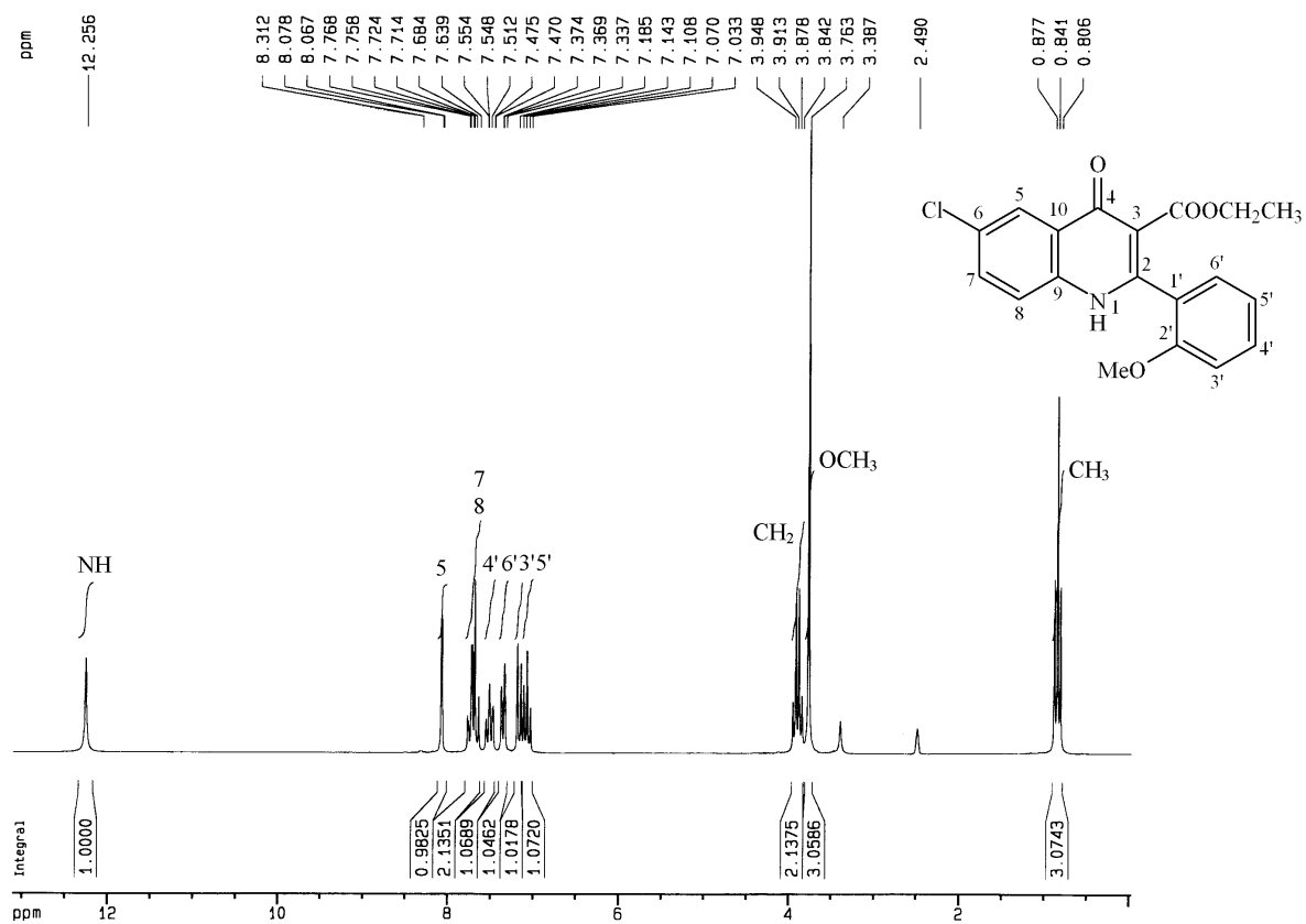
圖 33-3 化合物 33 之 ^1\text{H-NMR} ( \text{DMSO-}d_6 , 200 MHz)圖譜
