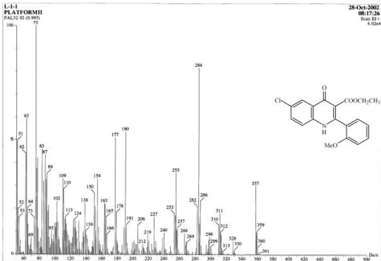
圖 33-1 化合物 33 之 MS 圖譜
