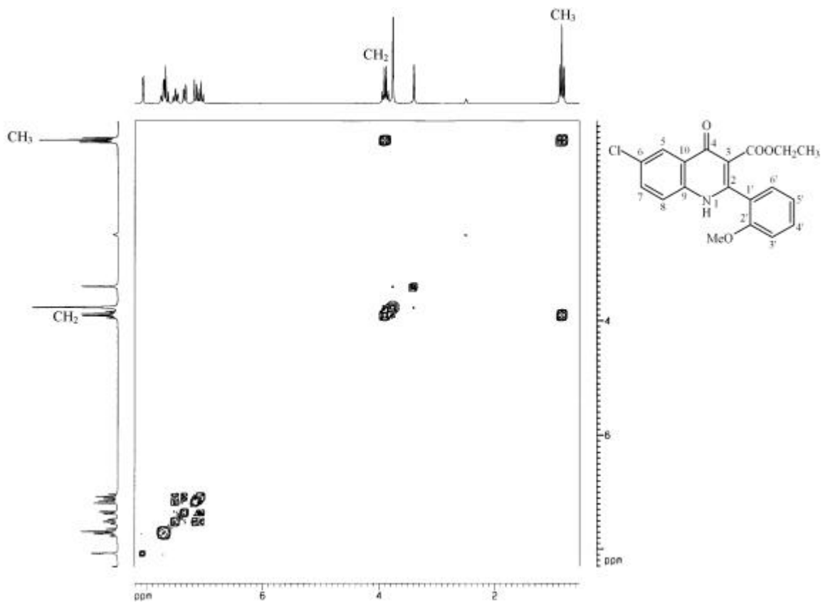
圖 33-4 化合物 33 之 ^1\text{H-}^1\text{H cosy} ( \text{DMSO-}d_6 , 200 MHz)圖譜
