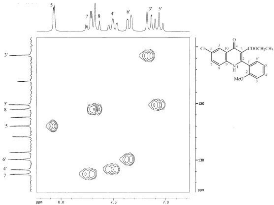
圖 33-8 化合物 33 之 HMQC (DMSO- d_6 , 200 MHz)圖譜
