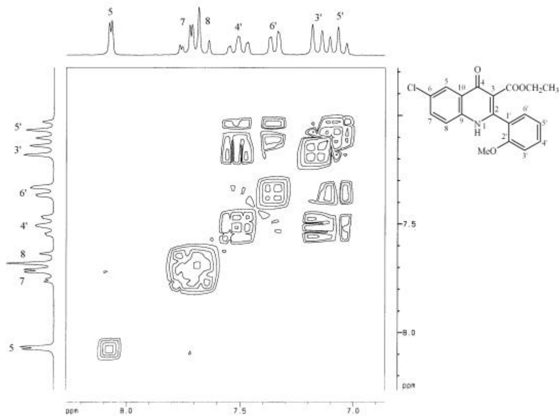
圖 33-5 化合物 33 之 ^1\text{H} - ^1\text{H} cosy (DMSO- d_6 , 200 MHz)圖譜
