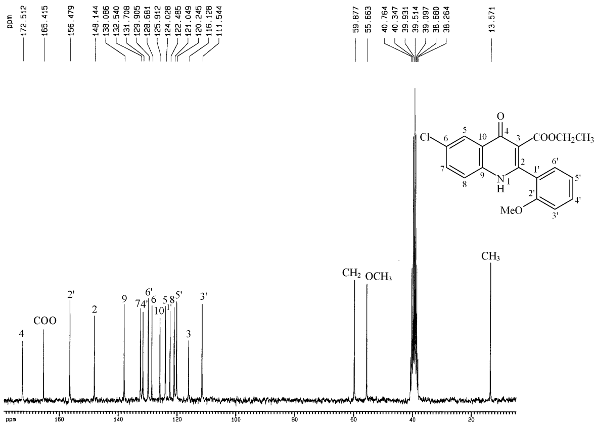
圖 33-6 化合物 33 之 ^{13}\text{C} -NMR (DMSO- d_6 , 50 MHz)圖譜
