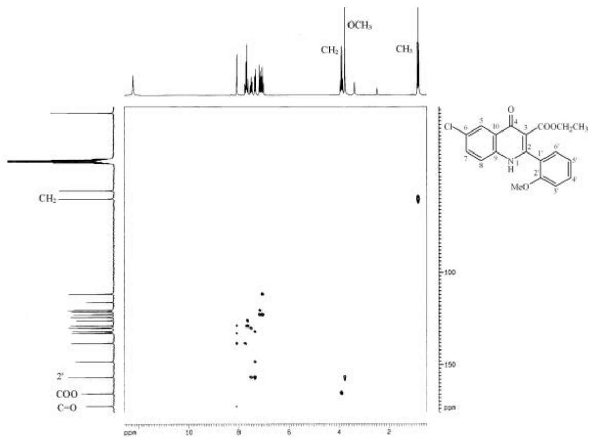
圖 33-9 化合物 33 之 HMBC (DMSO- d 6 , 200 MHz)圖譜
