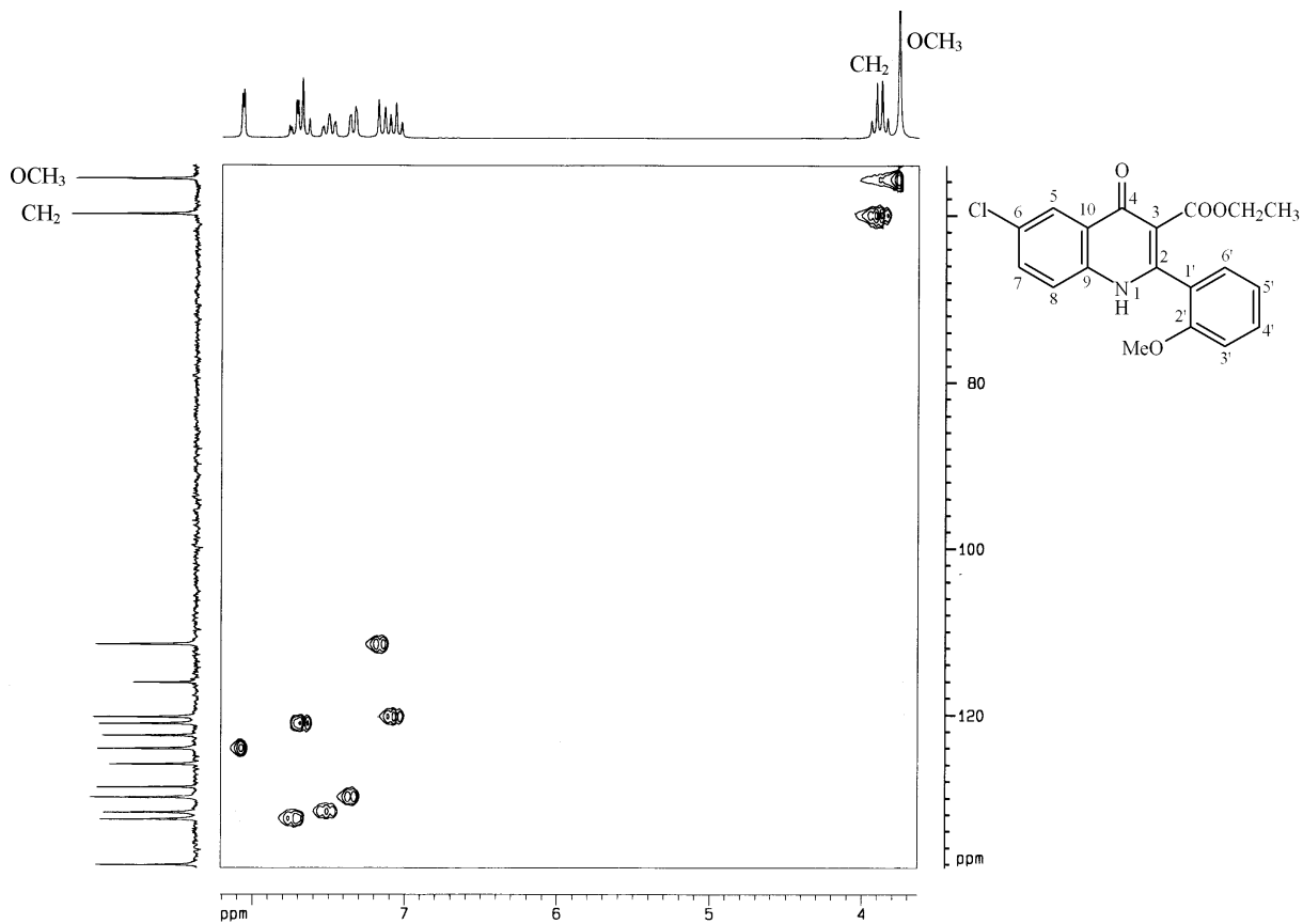
圖 33-7 化合物 33 之 HMQC (DMSO- d_6 , 200 MHz)圖譜
