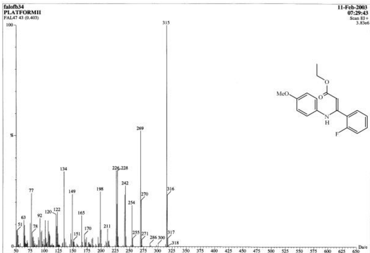
圖 29-1 化合物 29 之 MS 圖譜
