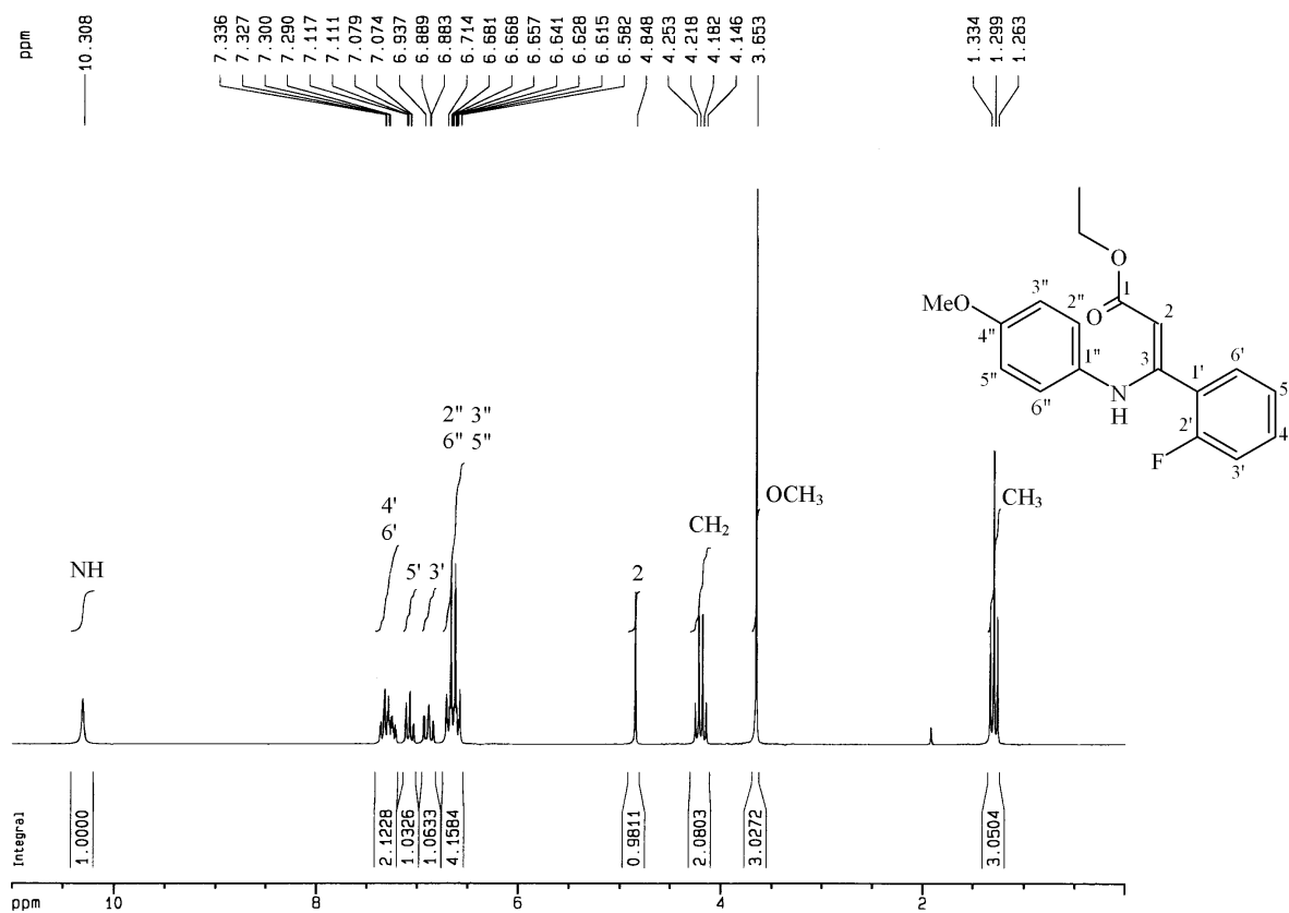
圖 29-3 化合物 29 之 1 H-NMR (Chloroform- d 1 , 200 MHz)圖譜
