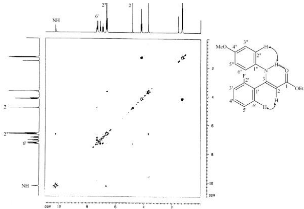
圖 29-6 化合物 29 之 NOESY (Chloroform- d_1 , 300 MHz)圖譜
