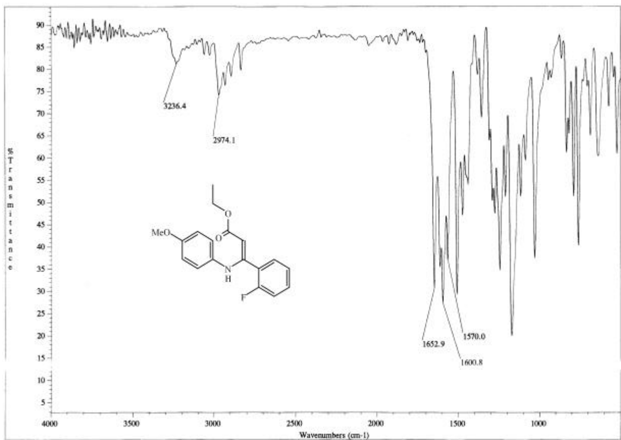
圖 29-2 化合物 29 之 IR 圖譜
