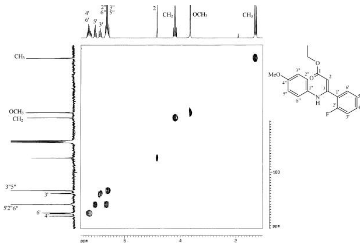
圖 29-5 化合物 29 之 HMQC (Chloroform- d_1 , 200 MHz)圖譜
