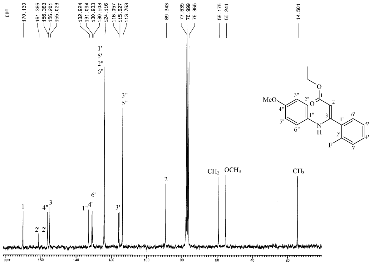
圖 29-4 化合物 29 之 13 C-NMR (Chloroform- d 1 , 50 MHz)圖譜
