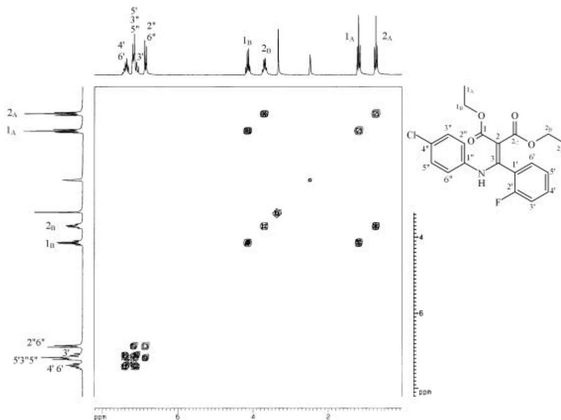
圖 26-5 化合物 26 之 ^1\text{H} - ^1\text{H} cosy (DMSO- d_6 , 50 MHz)圖譜
