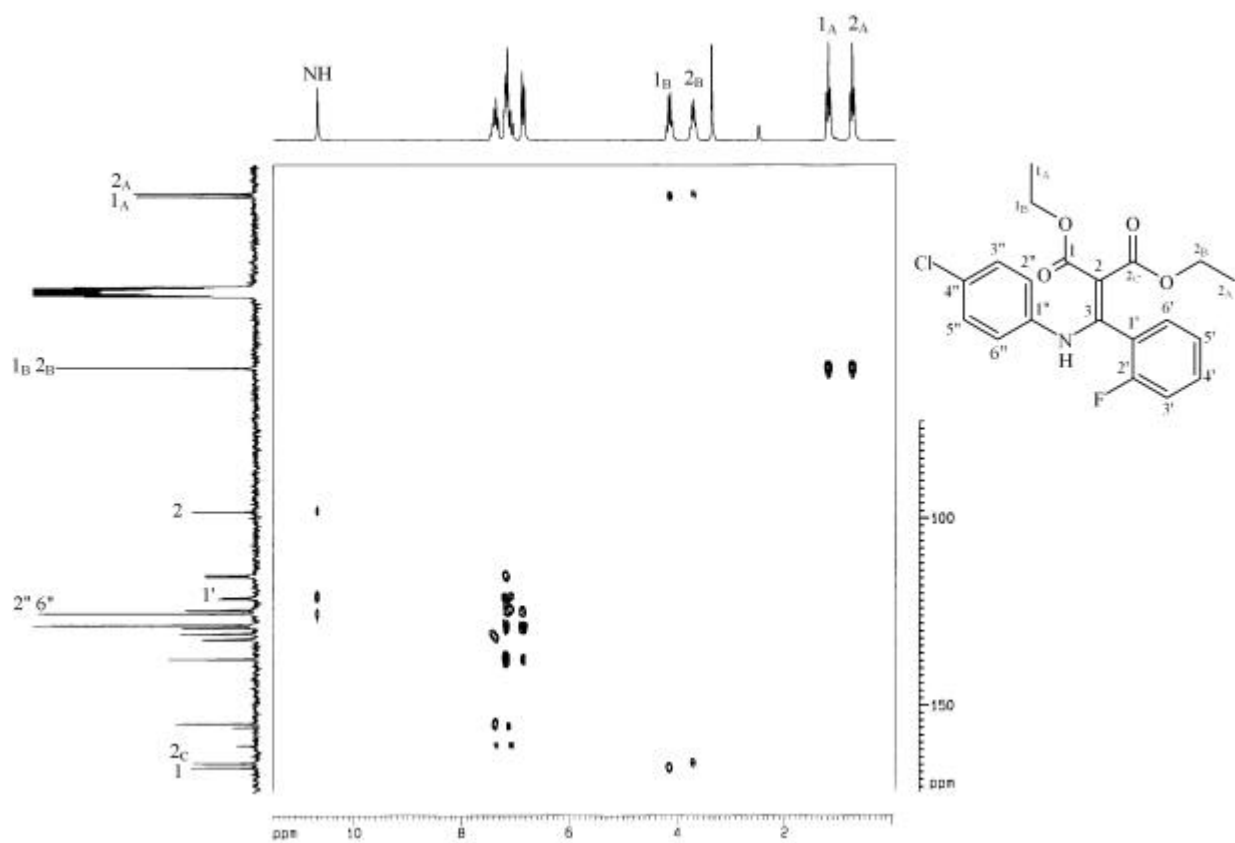
圖 26-8 化合物 26 之 HMBC (DMSO- d_6 , 200 MHz)圖譜
