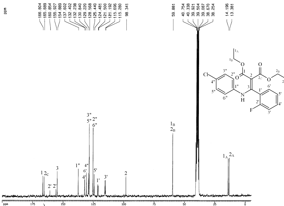
圖 26-6 化合物 26 之 ^{13}\text{C} -NMR (DMSO- d_6 , 200 MHz)圖譜
