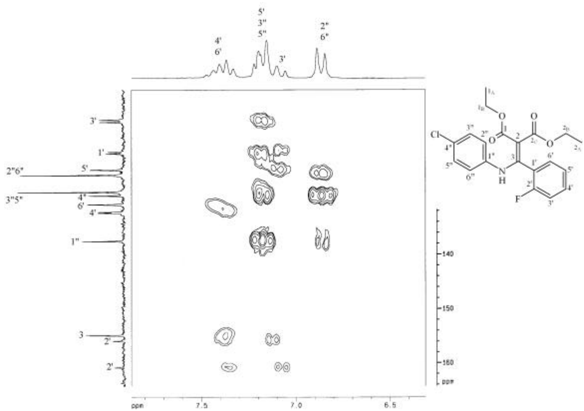
圖 26-9 化合物 26 之 HMBC (DMSO- d_6 , 200 MHz)圖譜
