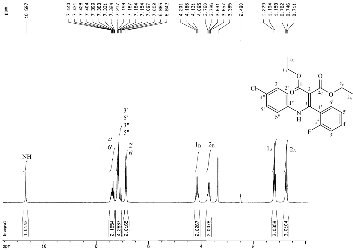
圖 26-3 化合物 26 之 1 H-NMR (DMSO- d 6 , 200 MHz)圖譜
