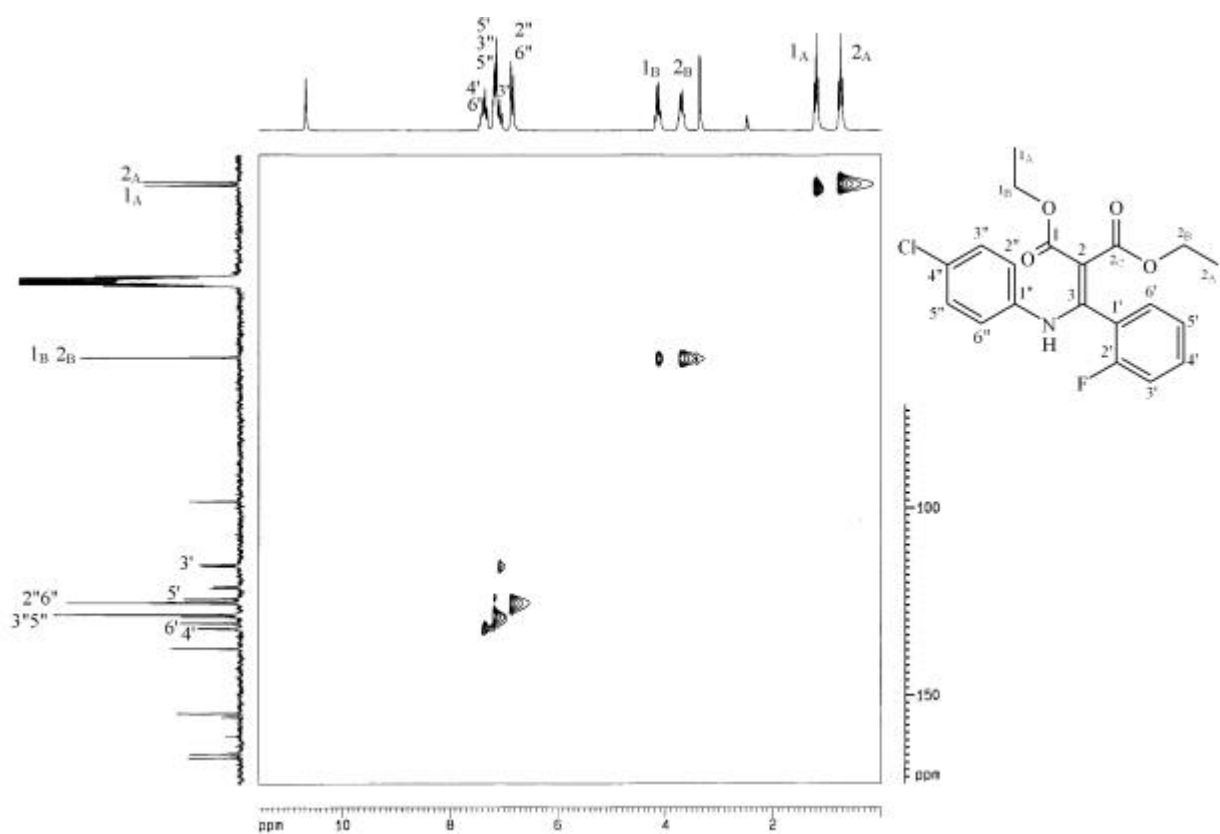
圖 26-7 化合物 26 之 HMQC (DMSO- d_6 , 200 MHz)圖譜
