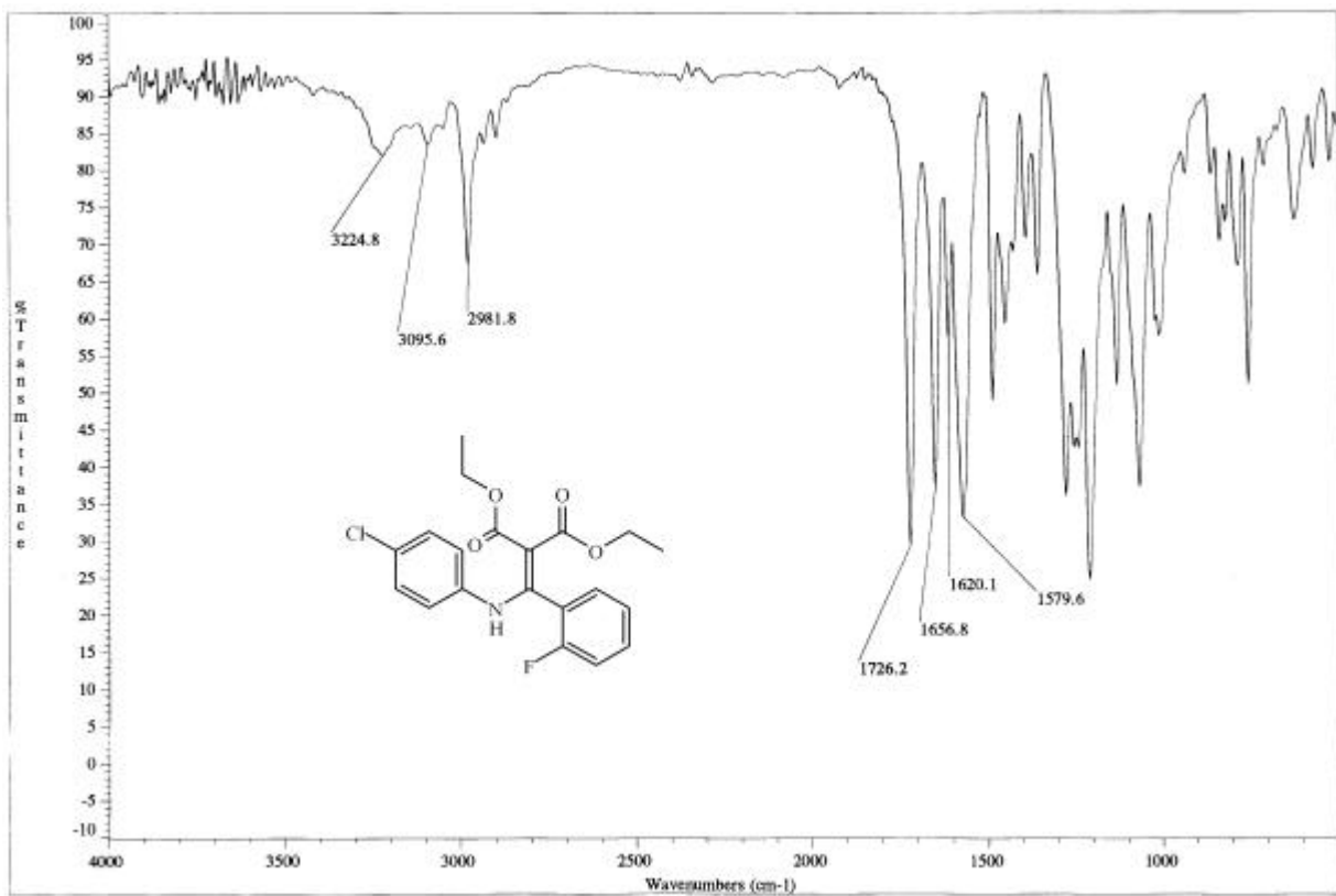
圖 26-2 化合物 26 之 IR 圖譜
