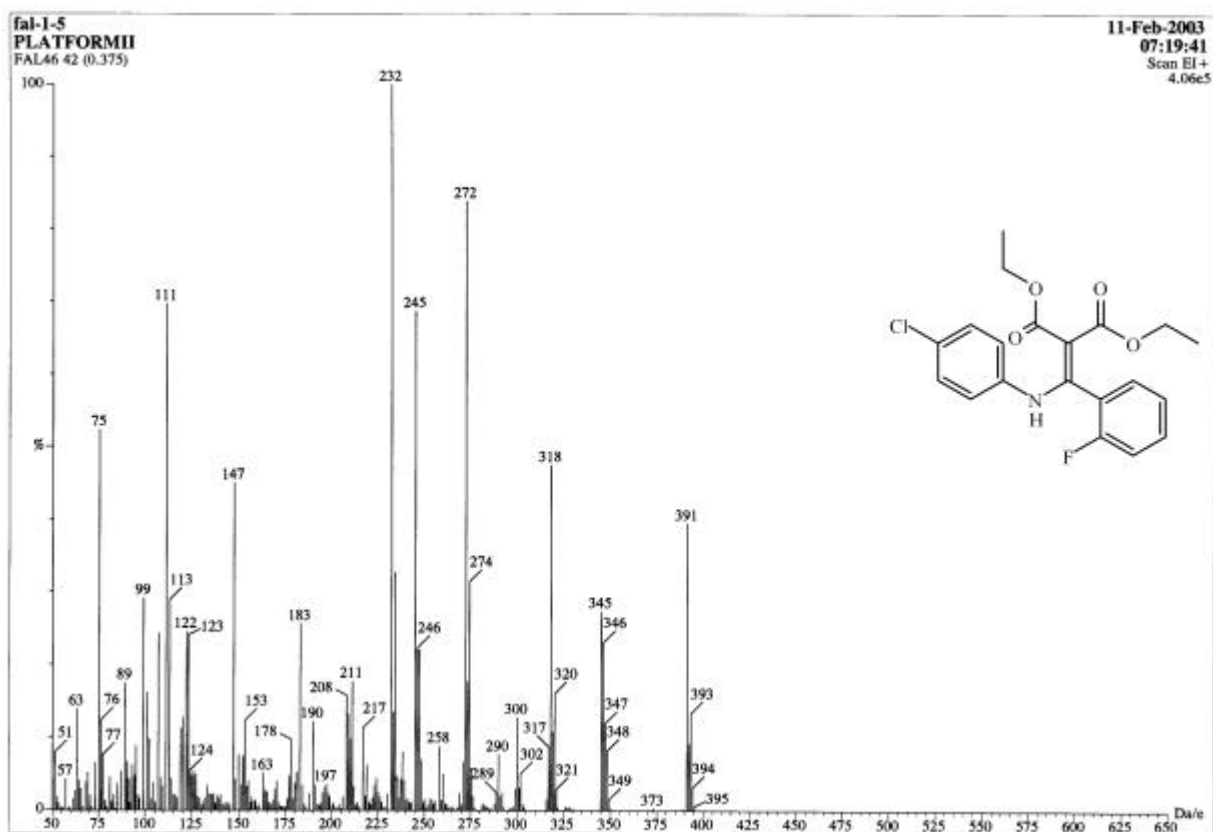
圖 26-1 化合物 26 之 MS 圖譜
