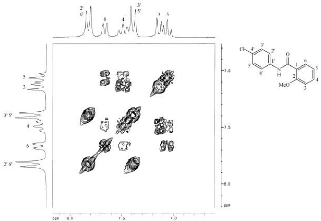
圖 13-4 化合物 13 之 ^1\text{H-}^1\text{H} cosy ( \text{DMSO-}d_6 , 200 MHz)圖譜
