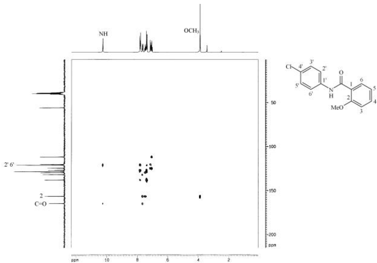
圖 13-7 化合物 13 之 HMBC (DMSO- d_6 , 200 MHz)圖譜
