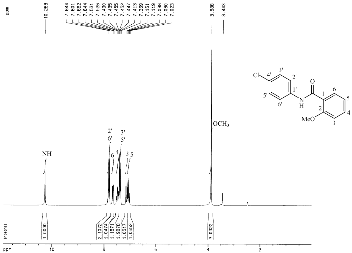
圖 13-3 化合物 13 之 ^1\text{H-NMR} ( \text{DMSO-}d_6 , 200 MHz)圖譜
