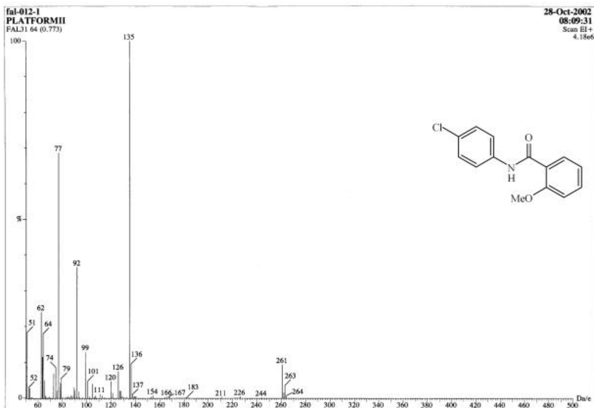
圖 13-1 化合物 13 之 MS 圖譜
