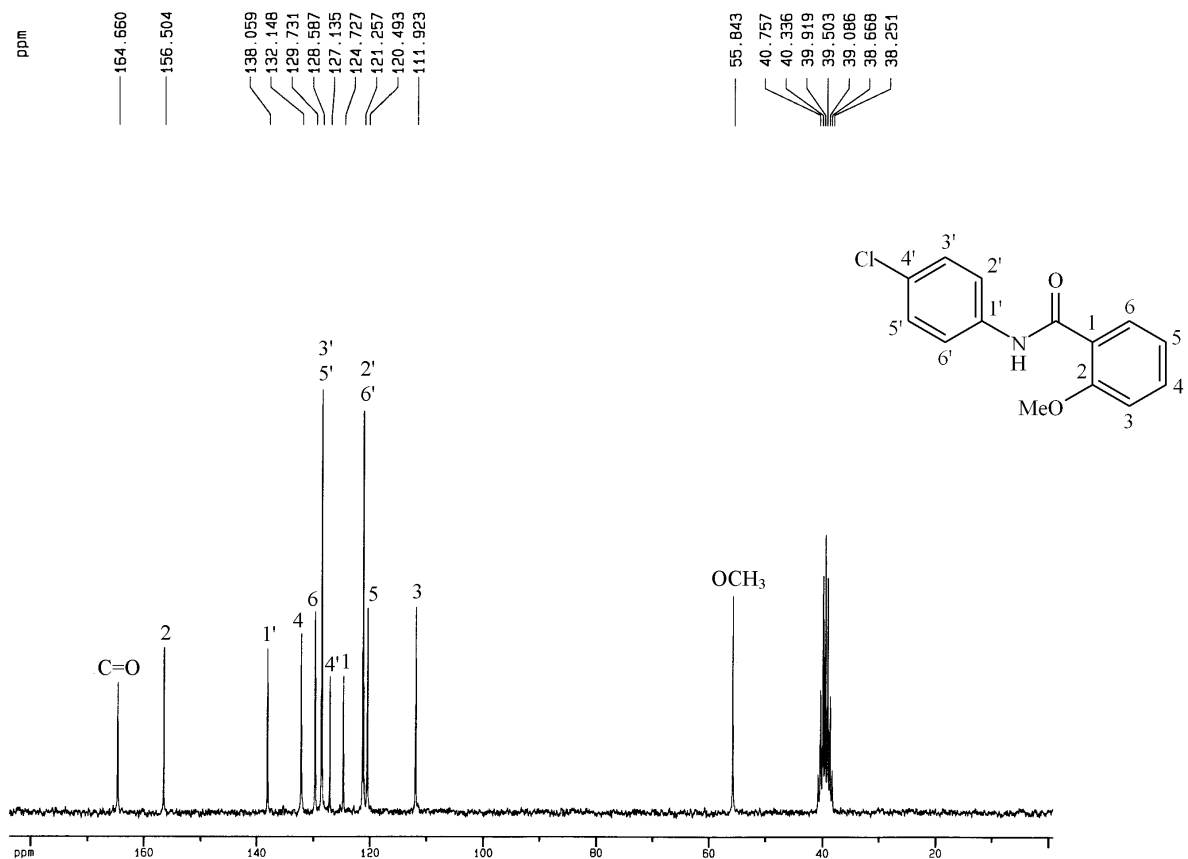
圖 13-5 化合物 13 之 ^{13}\text{C-NMR} (DMSO- d_6 , 50 MHz)圖譜
