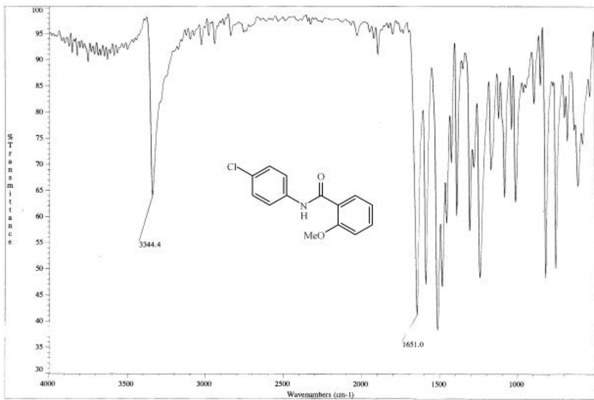
圖 13-2 化合物 13 之 IR 圖譜
