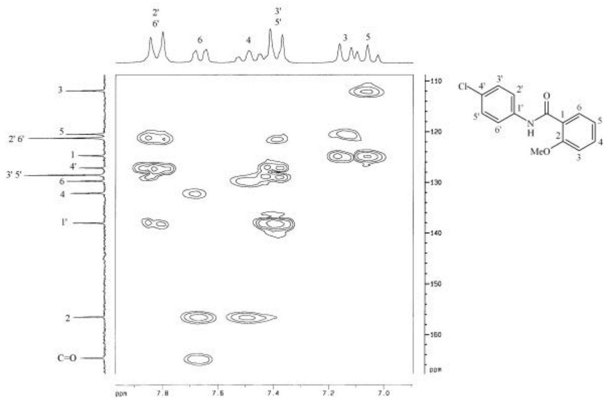
圖 13-8 化合物 13 之 HMBC (DMSO- d_6 , 200 MHz)圖譜
