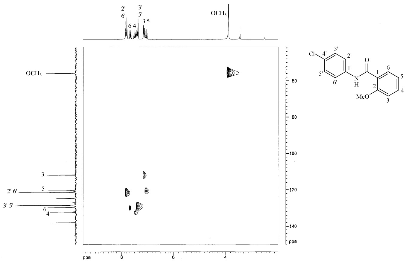
圖 13-6 化合物 13 之 HMBC (DMSO- d_6 , 200 MHz)圖譜
