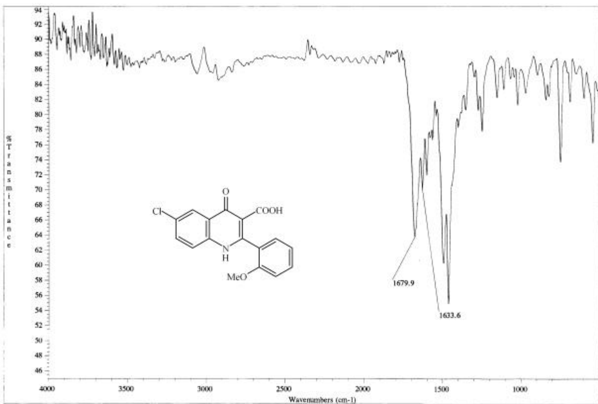
圖 47-2 化合物 47 之 IR 圖譜
