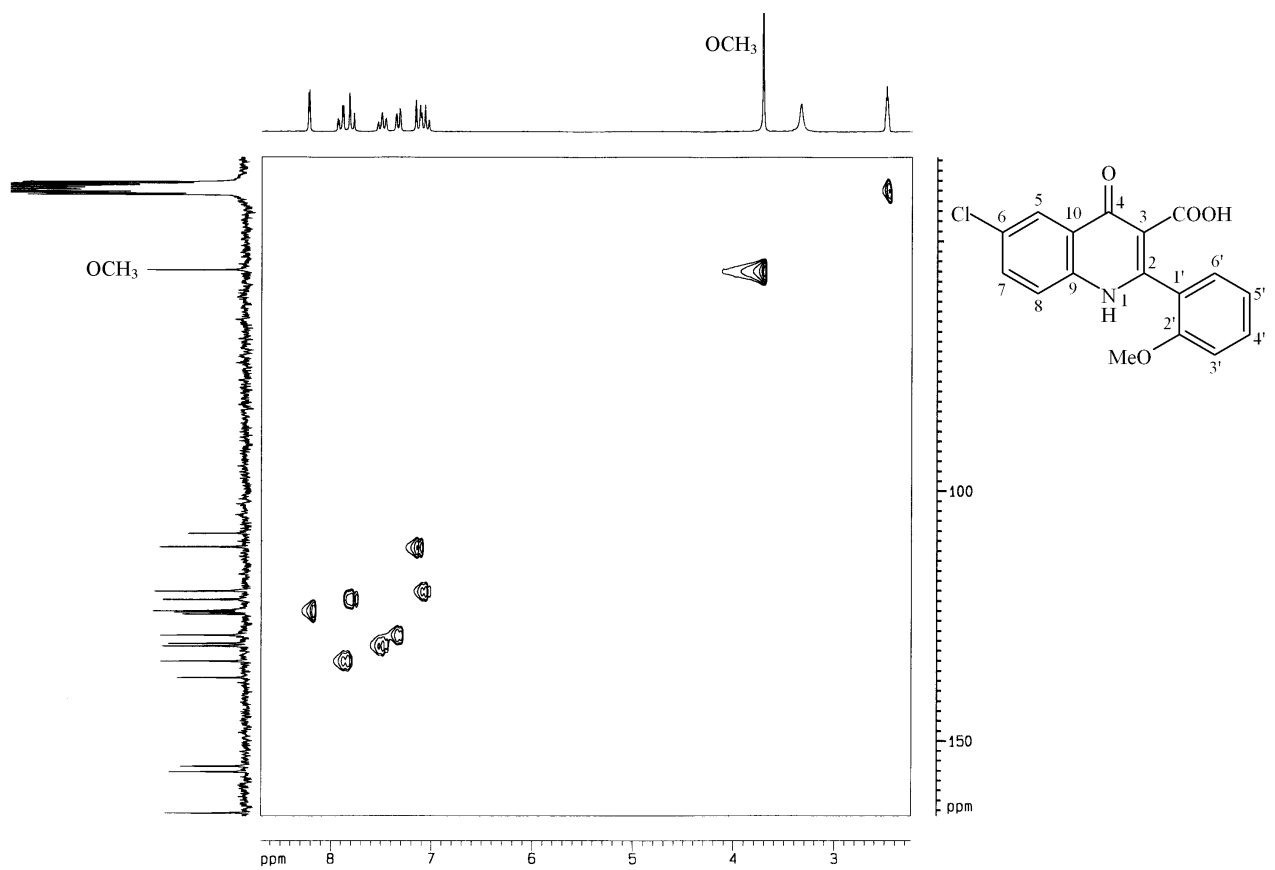
圖 47-6 化合物 47 之 HMQC ( \text{DMSO-}d_6 , 200 MHz)圖譜
