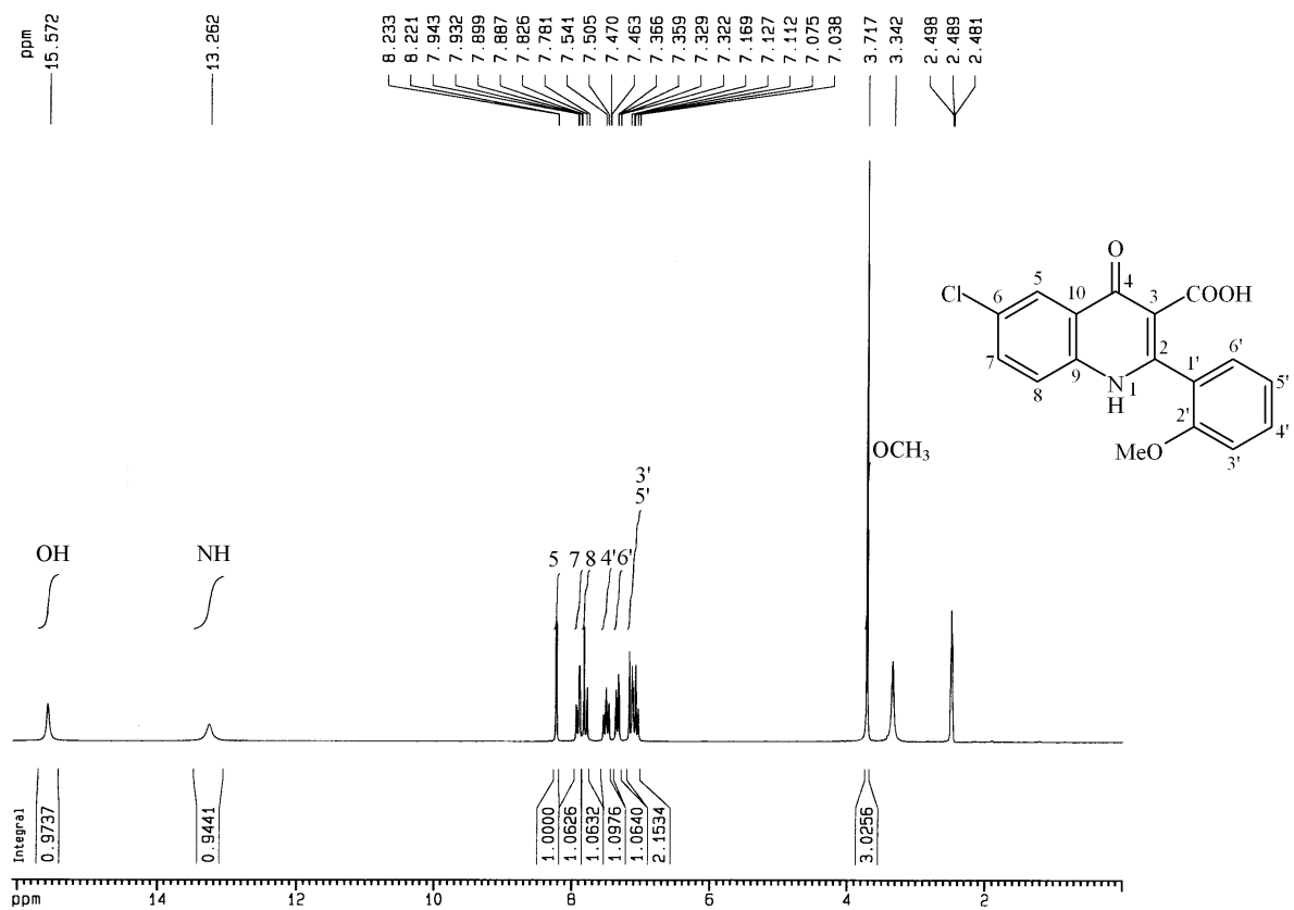
圖 47-3 化合物 47 之 ^1\text{H-NMR} (DMSO- d_6 , 200 MHz)圖譜
