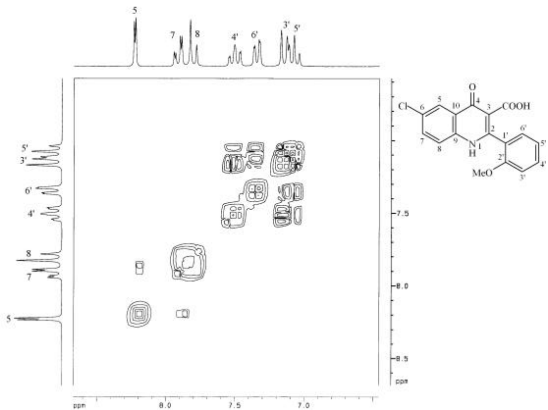
圖 47-4 化合物 47 之 ^1\text{H-}^1\text{H} cosy (DMSO- d_6 , 200 MHz)圖譜
