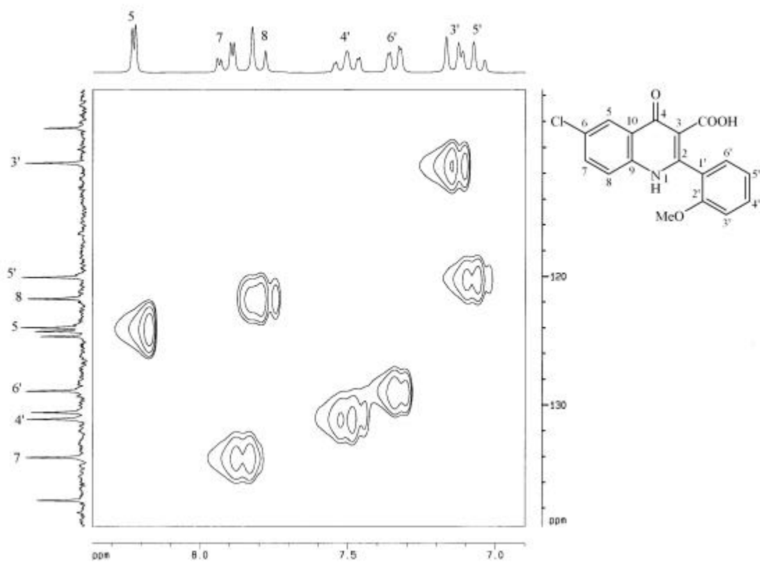
圖 47-7 化合物 47 之 HMQC (DMSO- d_6 , 200 MHz)圖譜
