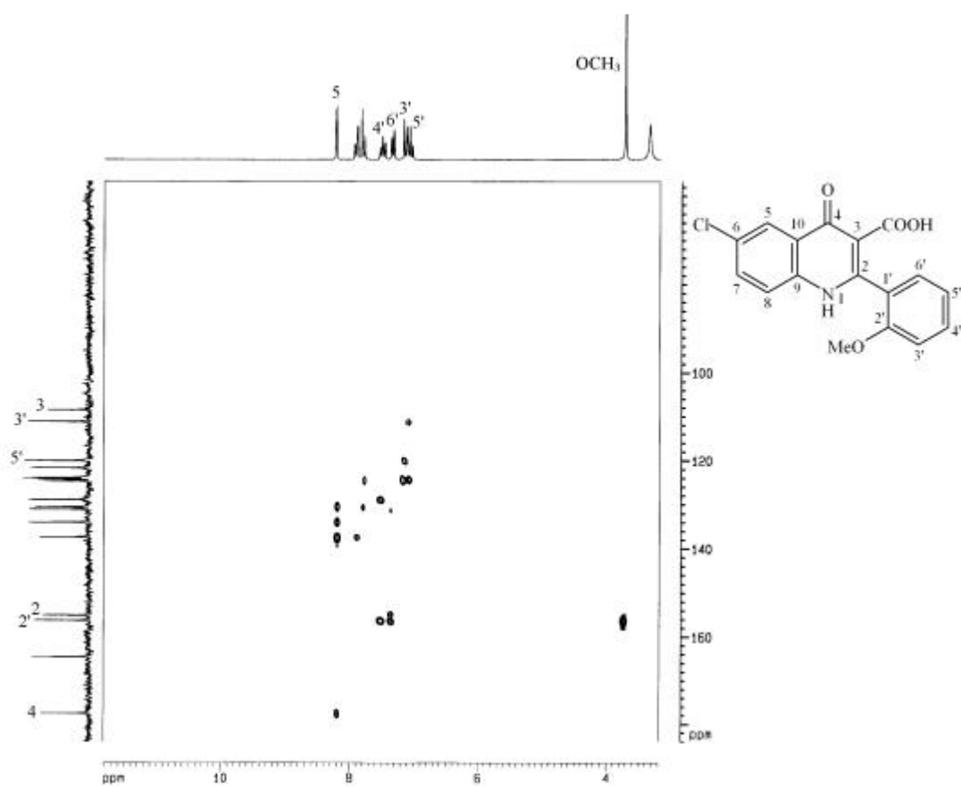
圖 47-8 化合物 47 之 HMBC (DMSO- d_6 , 200 MHz)圖譜
