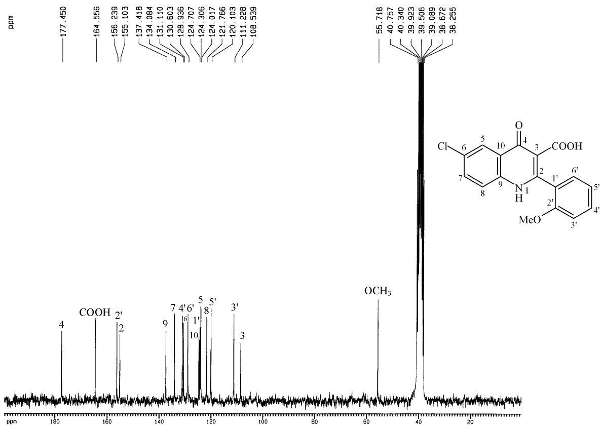
圖 47-5 化合物 47 之 ^{13}\text{C-NMR} ( \text{DMSO-}d_6 , 50 MHz)圖譜
