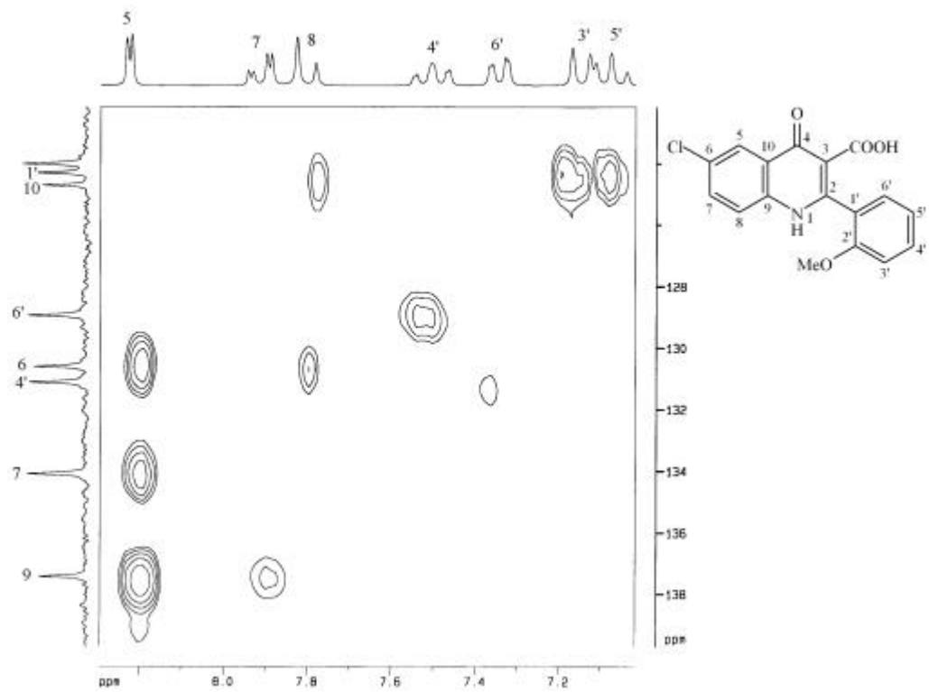
圖 47-9 化合物 47 之 HMBC (DMSO- d_6 , 200 MHz)圖譜
