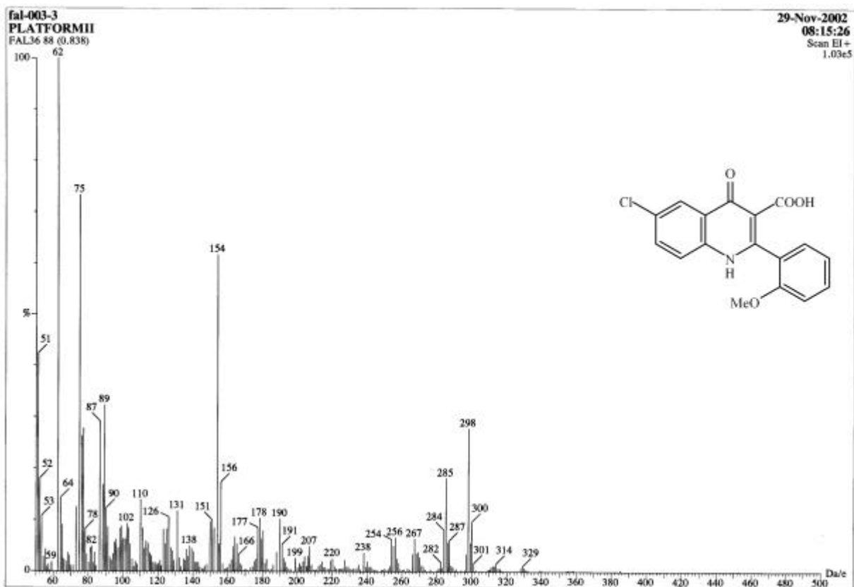
圖 47-1 化合物 47 之 MS 圖譜
