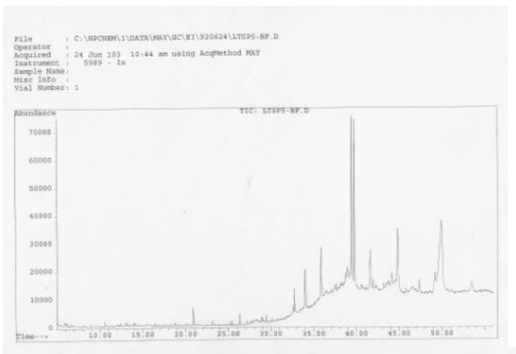
圖 21 LJSP5-BF 毛忍冬幼蕾(埔里產)氣相層析圖
