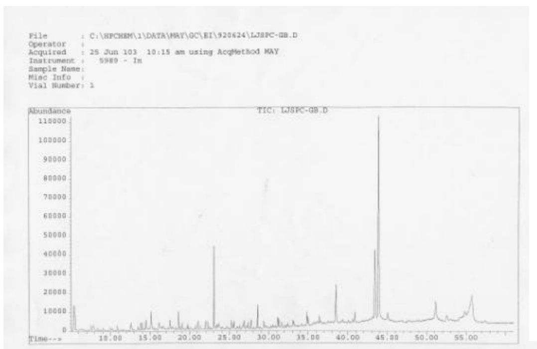
圖 26 LJSPC-GB 毛忍冬綠薔(田尾產)氣相層析圖
