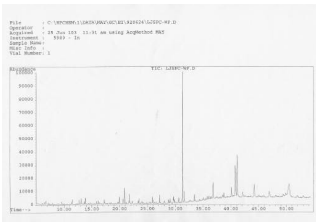
圖 27 LJSPC-WF毛忍冬白花(田尾產)氣相層析圖
