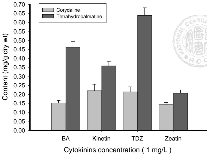
圖 40. Cytokinins 對植物生長調節劑癒合組織產生 corydaline 及 tetrahydropalmatine 之影響
