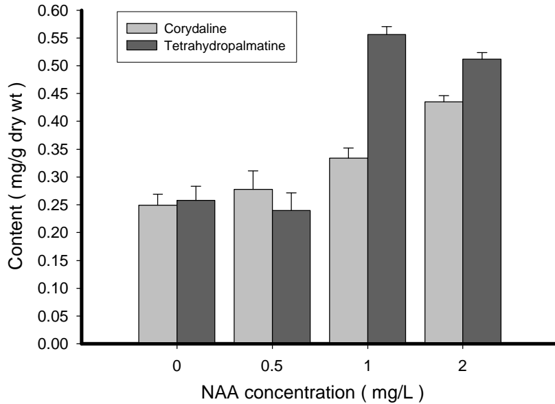
圖 39. NAA 對癒合組織產生 corydaline 及 tetrahydropalmatine 之影響
