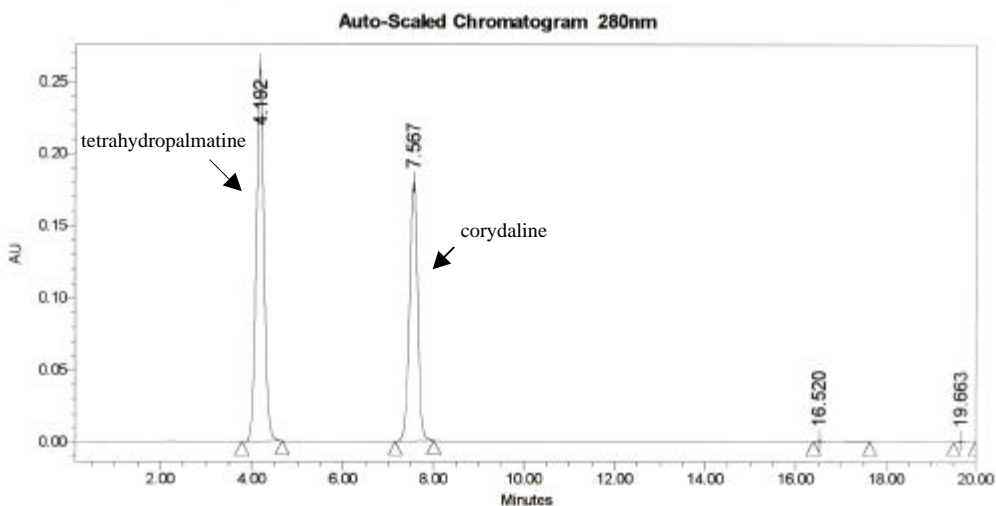
圖 11. 延胡索甲素 (corydaline) 及乙素 (tetrahydropalmatine) 標準品 HPLC 圖譜
