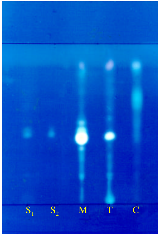
圖 10. 延胡索檢品之 TLC 定性分析
