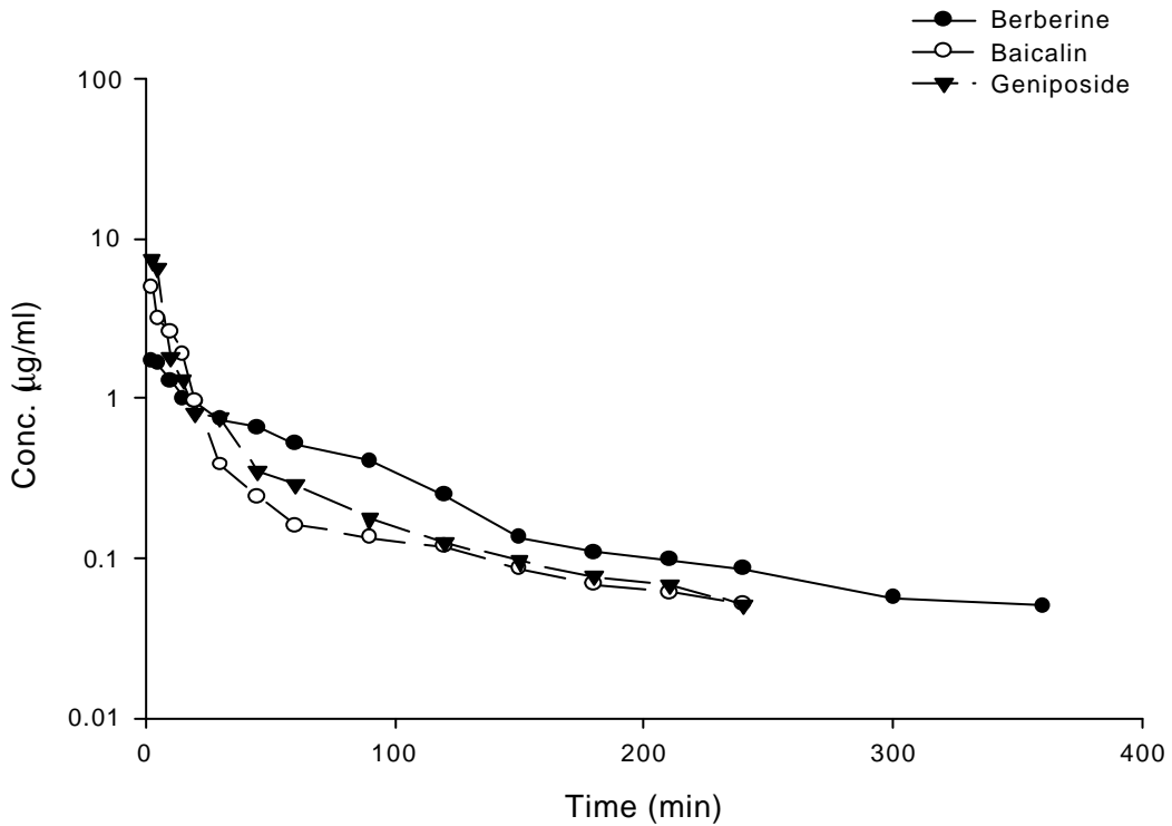
Figure 19 家兔(No 1, No 2)靜脈注射黃連解毒湯注射液後, Berberine、Baicalin 及 Geniposide 之血漿中濃度-時間曲線圖。
