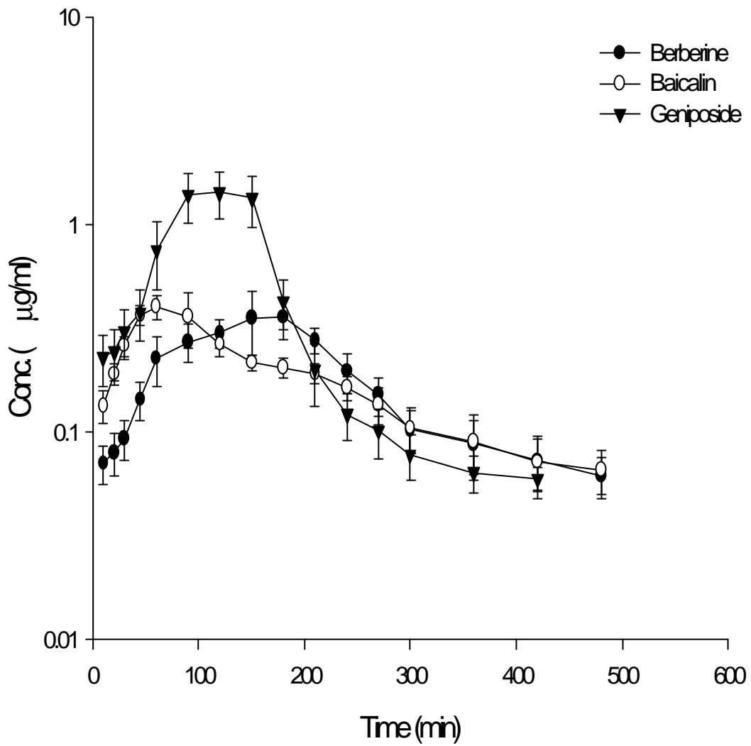
Figure 26 六隻家兔口服黃連解毒湯口服液後，Berberine、Baicalin 及 Geniposide 之血漿中平均濃度-時間曲線圖。
