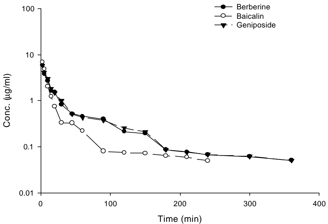
Figure 17 家兔(No 5, No 6)靜脈注射三種指標成分標準品 Berberine、Baicalin 及 Geniposide 後之血漿中濃度-時間曲線圖。
