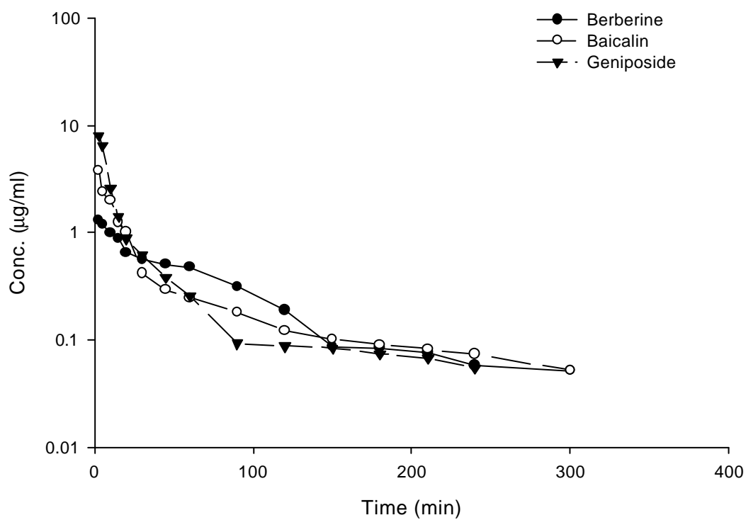
Figure 20 家兔(No 3, No 4)靜脈注射黃連解毒湯注射液後, Berberine、Baicalin 及 Geniposide 之血漿中濃度-時間曲線圖。
