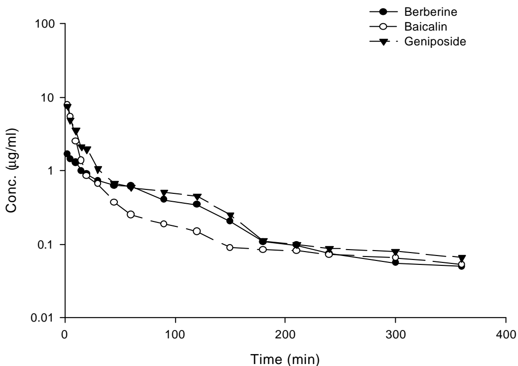
Figure 16 家兔(No 3, No 4)靜脈注射三種指標成分標準品 Berberine、Baicalin 及 Geniposide 後之血漿中濃度-時間曲線圖。
