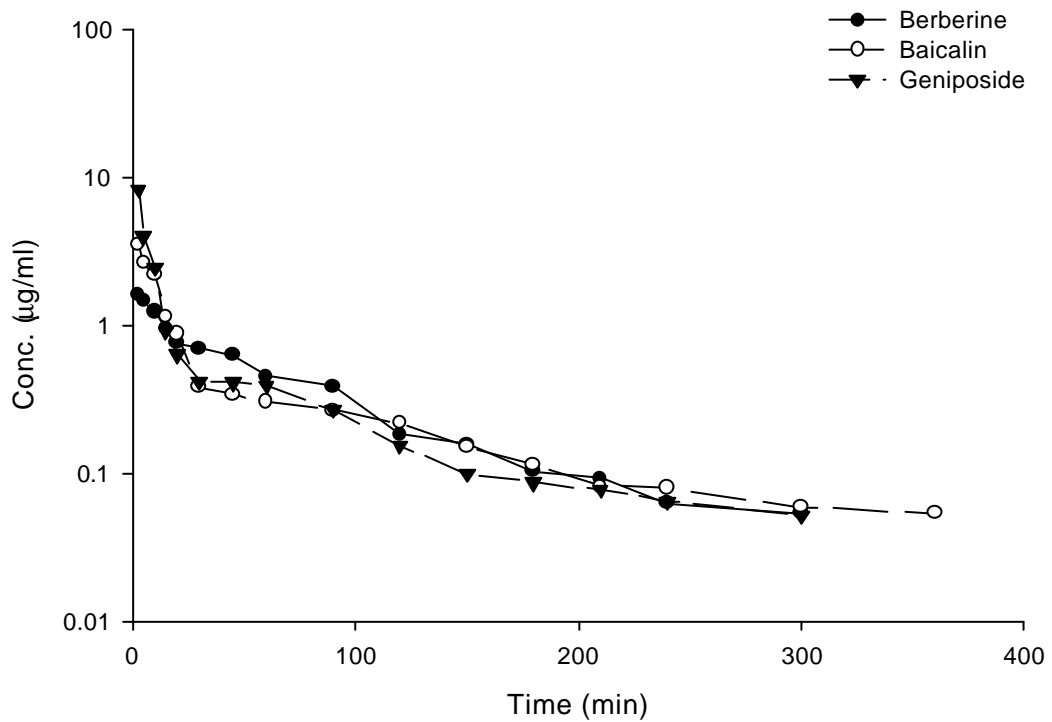
Figure 21 家兔(No 5, No 6)靜脈注射黃連解毒湯注射液後, Berberine、Baicalin 及 Geniposide 之血漿中濃度-時間曲線圖。
