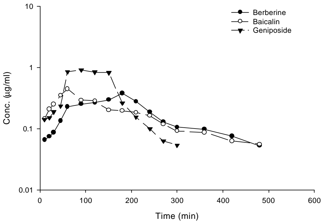
Figure 25 家兔(No 5, No 6)口服黃連解毒湯口服液後, Berberine、Baicalin 及 Geniposide 之血漿中濃度-時間曲線圖。
