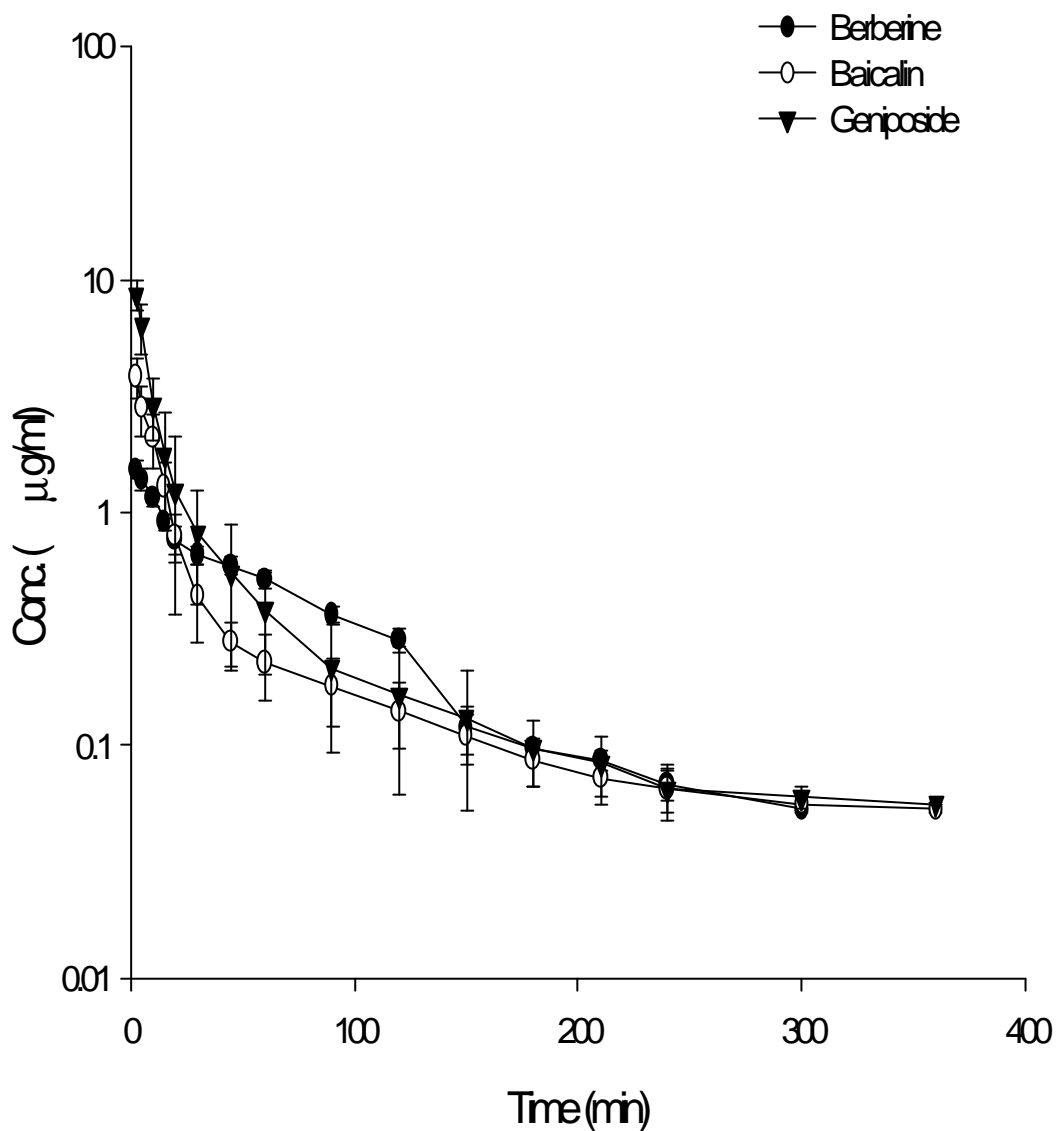
Figure 22 六隻家兔靜脈注射黃連解毒湯注射液後 Berberine、Baicalin 及 Geniposide 之平均血漿中濃度-時間曲線圖。
