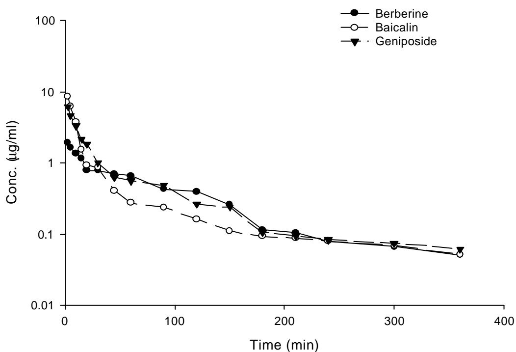
Figure 15 家兔(No 1, No 2)靜脈注射三種指標成分標準品 Berberine、Baicalin 及 Geniposide 後之血漿中濃度-時間曲線圖。
