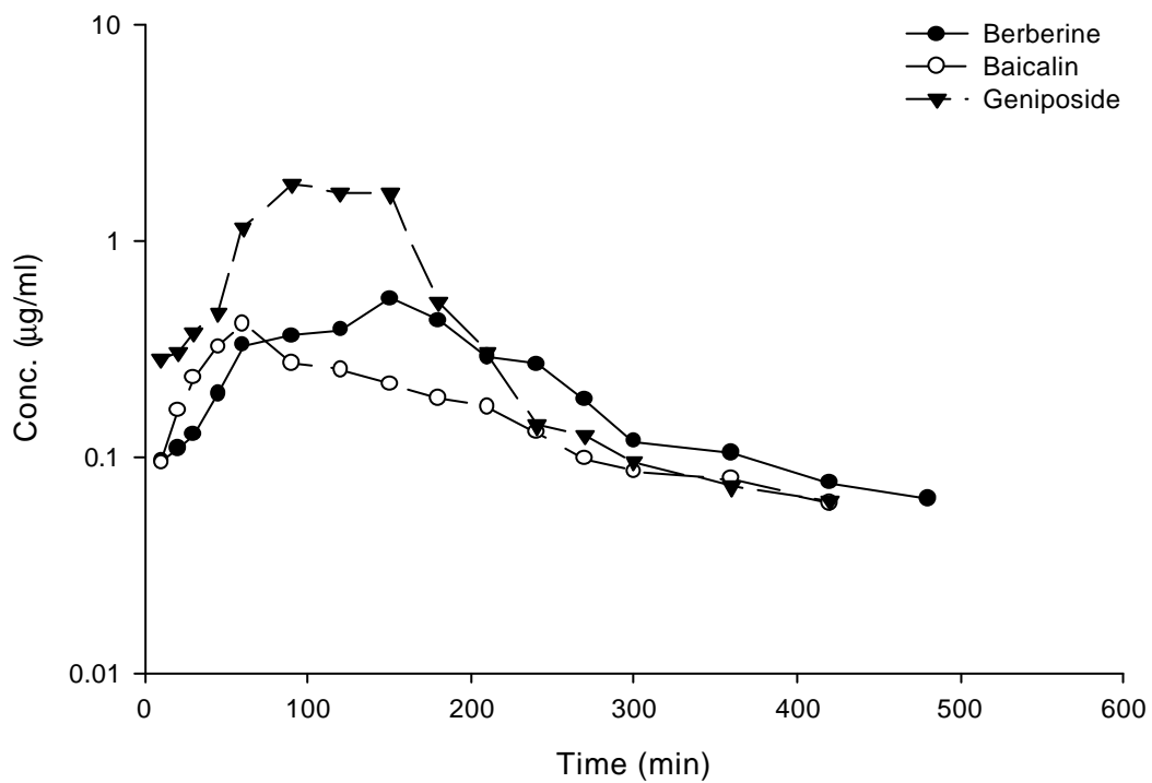
Figure 23 家兔(No 1, No 2)口服黃連解毒湯口服液後, Berberine、Baicalin 及 Geniposide 之血漿中濃度-時間曲線圖。
