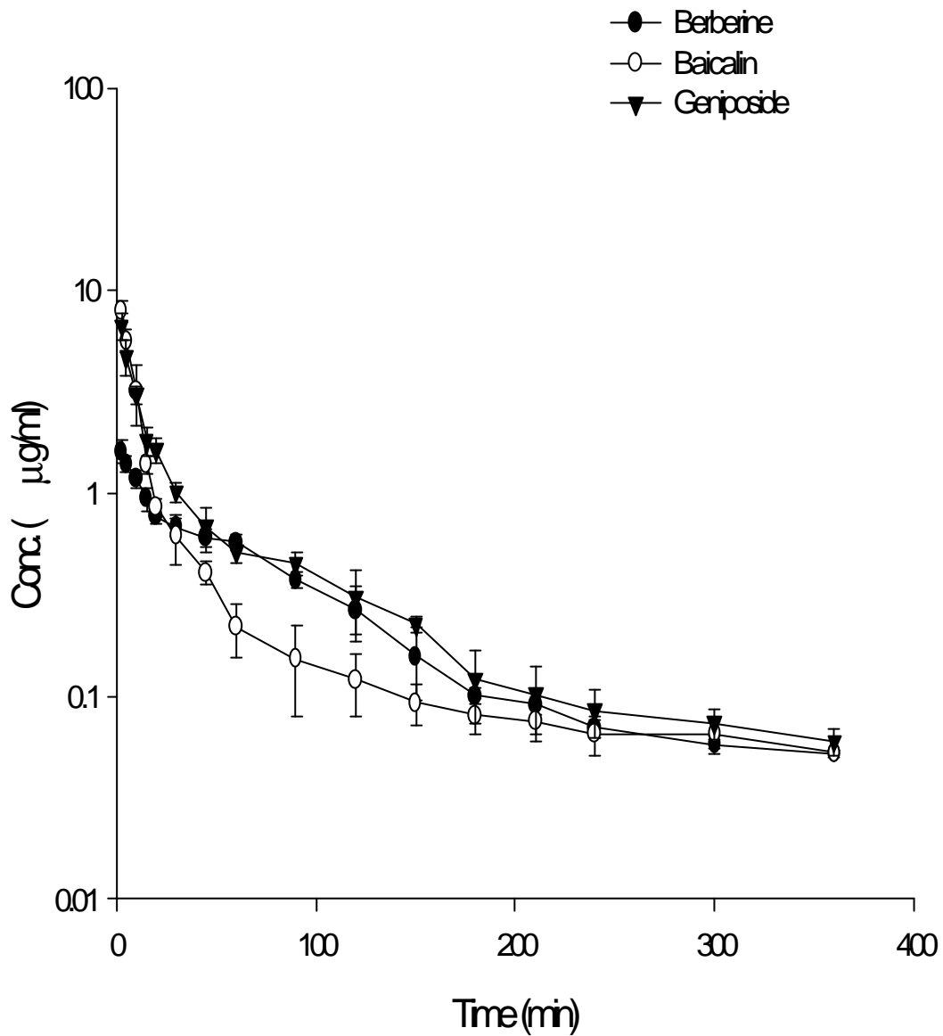
Figure 18 六隻家兔靜脈注射三種指標成分標準品 Berberine、Baicalin 及 Geniposide 後之平均血漿中濃度-時間曲線圖。
