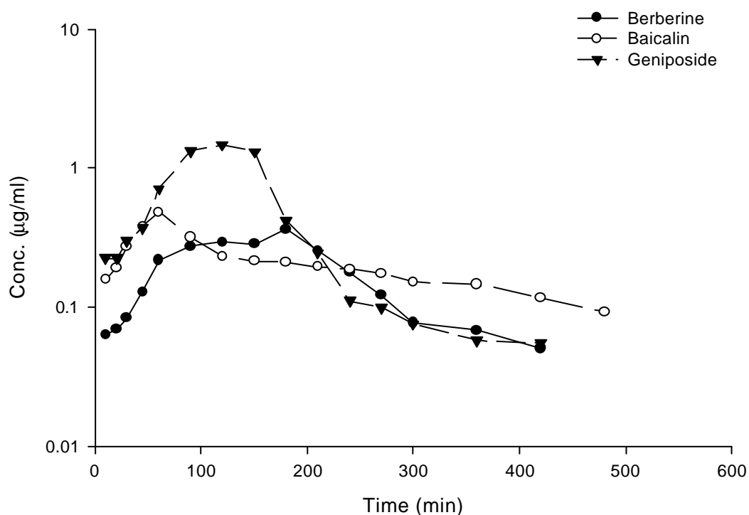
Figure 24 家兔(No 3, No 4)口服黃連解毒湯口服液後, Berberine、Baicalin 及 Geniposide 之血漿中濃度-時間曲線圖。
