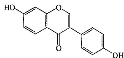
大豆苷元(daidzein)
