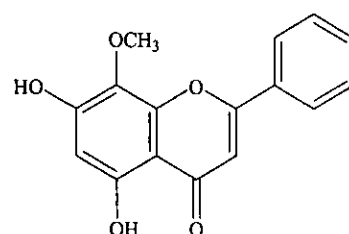
漢黃芩素(wogonin)
