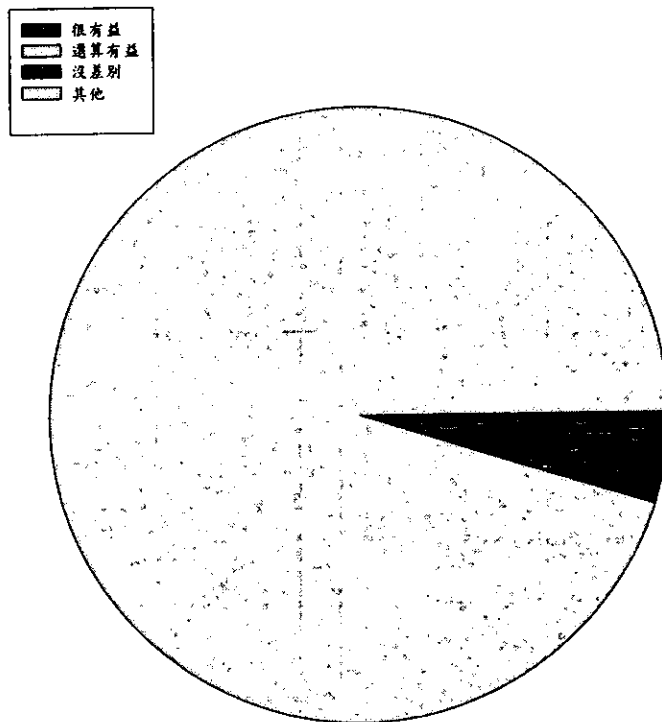
圖 22 對於 NMR 所作統計方法，多變數分析(Multiple variance analysis)中的 Principal component analysis(PCA)的統計方法的概念
