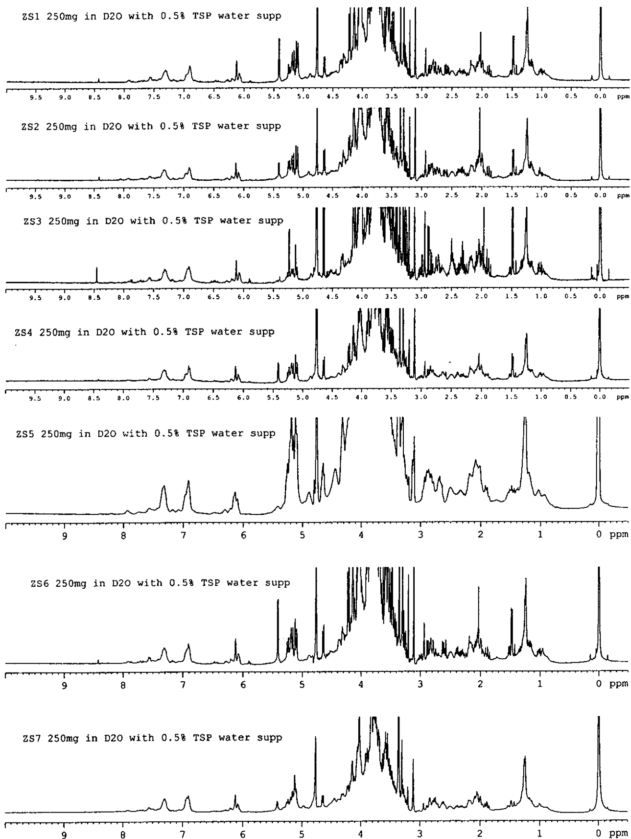
圖 7 枳實的 NMR 圖譜
