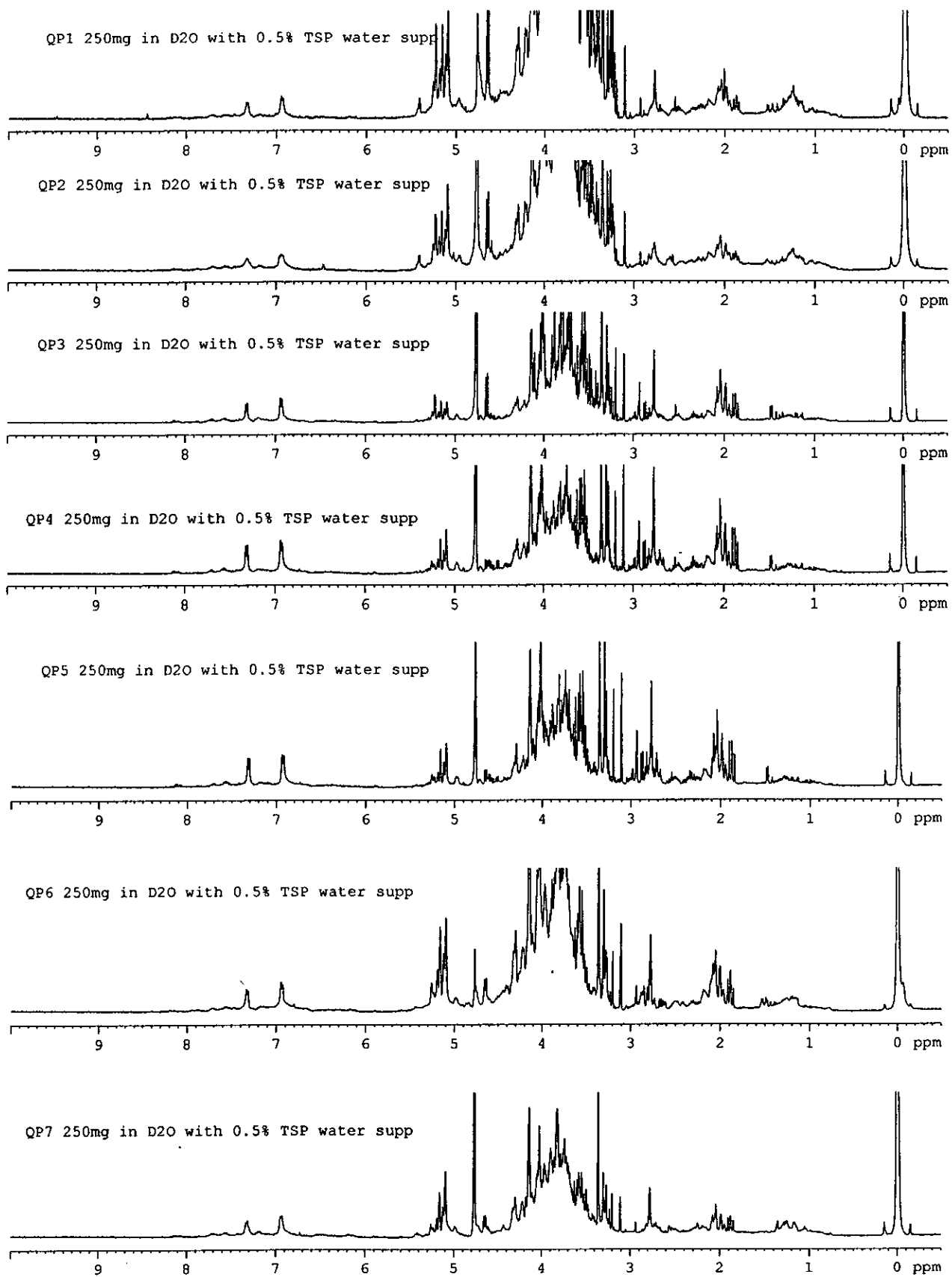
圖 5 青皮的 NMR 圖譜
