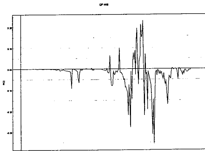
圖 13-2 青皮的 loading plot PC2
