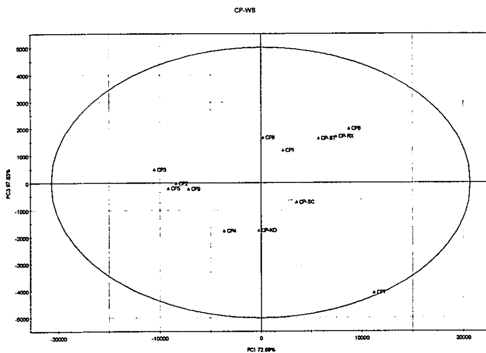
圖 8-1 陳皮的 score plot PC1 與 PC2
