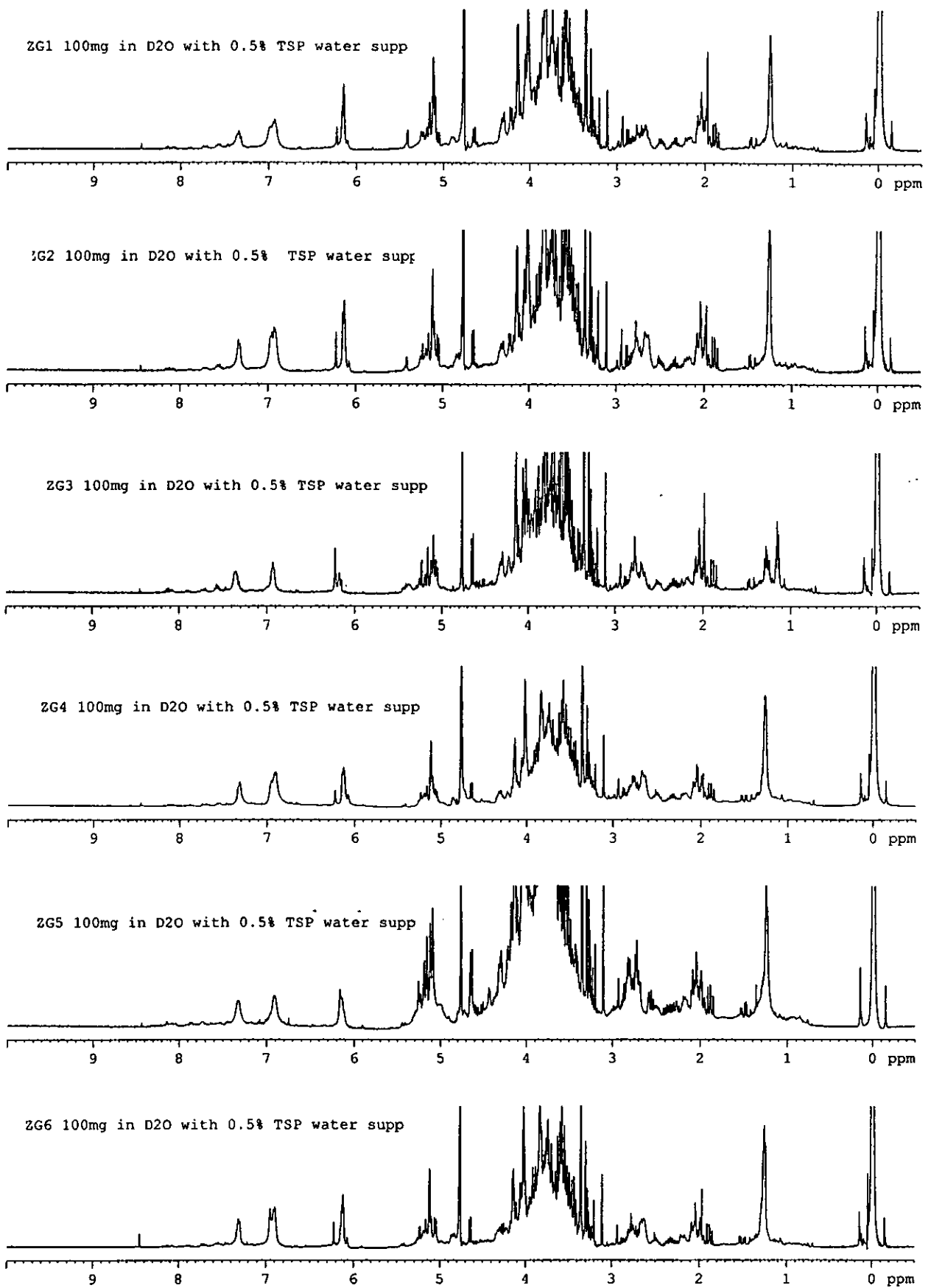
圖 6 枳殼的 NMR 圖譜
