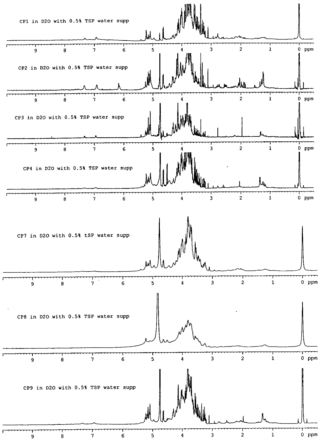
圖3 陳皮的NMR圖譜
