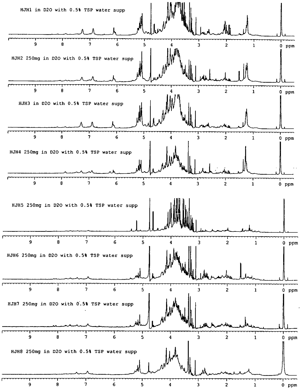
圖 4 橘紅的 NMR 圖譜
